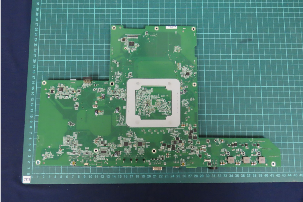
(31) EUT Photo
