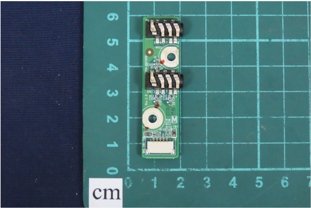
(108)EUT Photo
