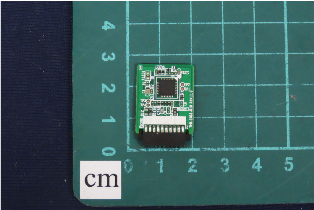
(107)EUT Photo
