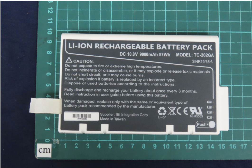
(125)EUT Photo
