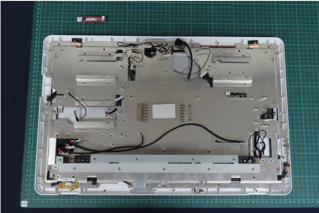
(117)EUT Photo
