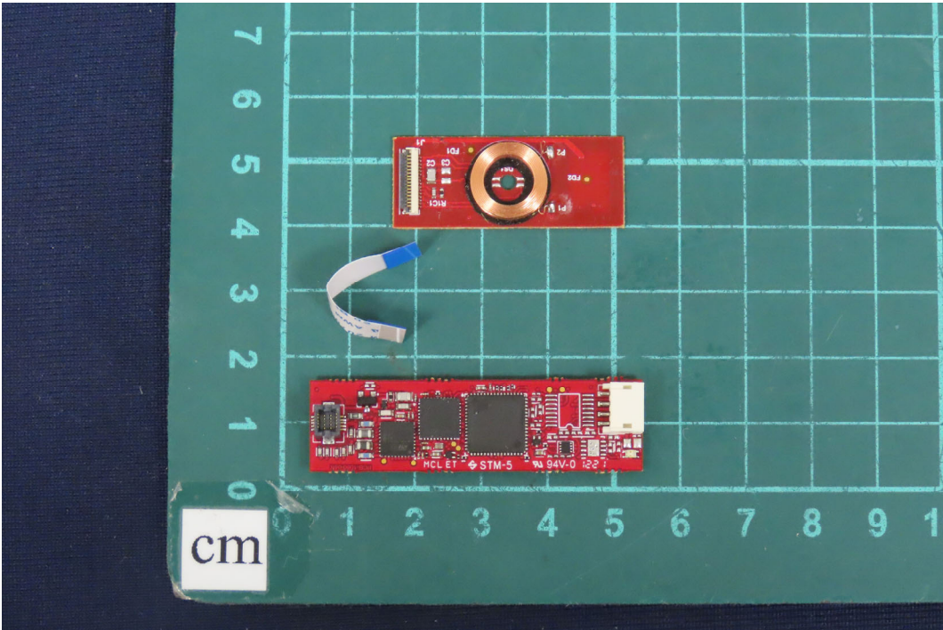
(119)EUT Photo
