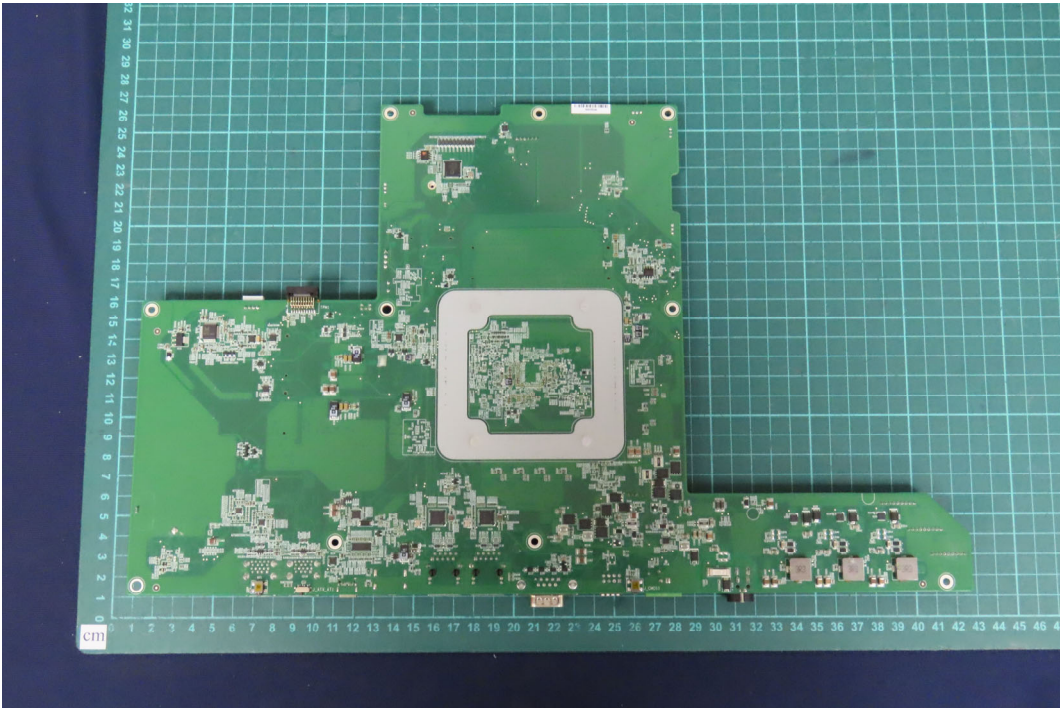
(113)EUT Photo
