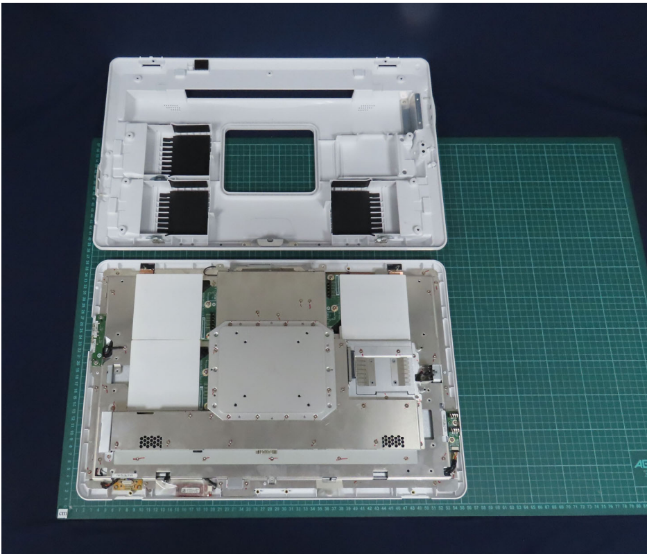
(128)EUT Photo
