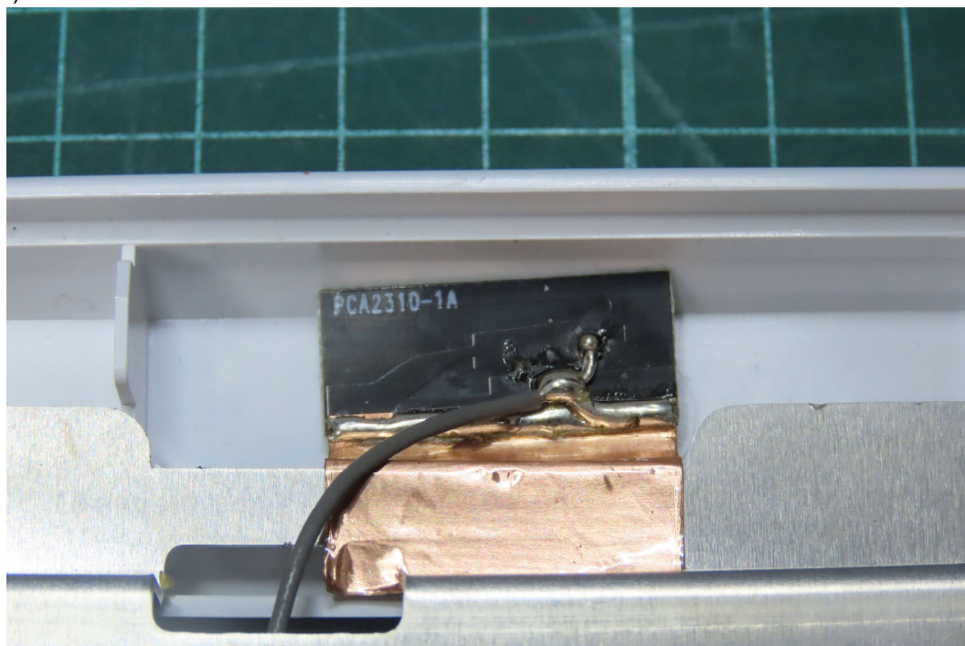
(116)EUT Photo
