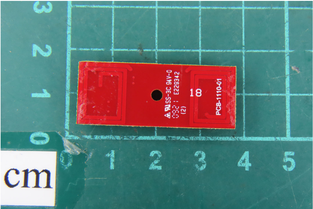
(123)EUT Photo
