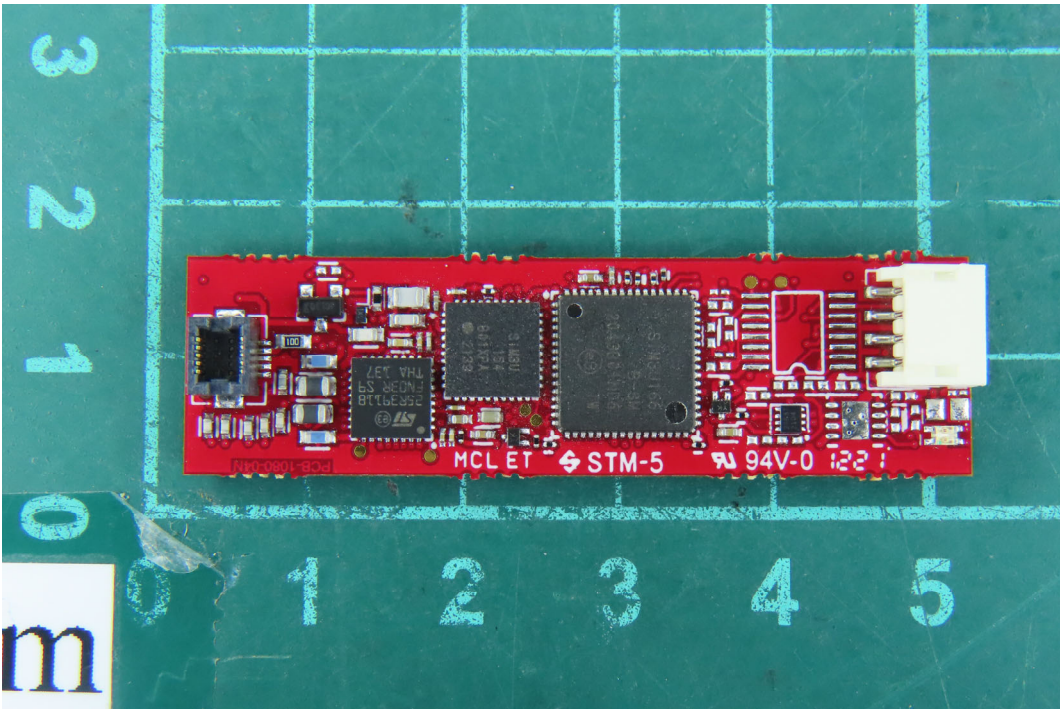
(120)EUT Photo
