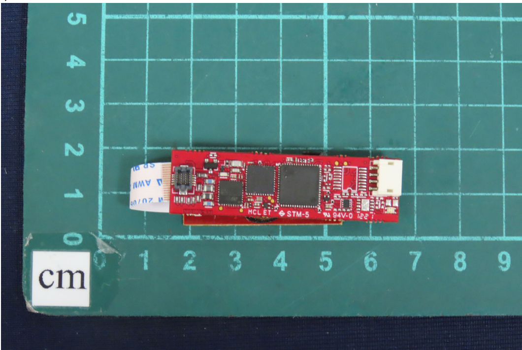
(118)EUT Photo
