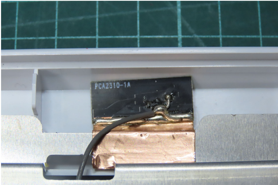
(157)EUT Photo
