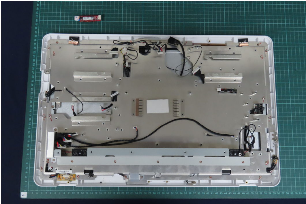
(158)EUT Photo
