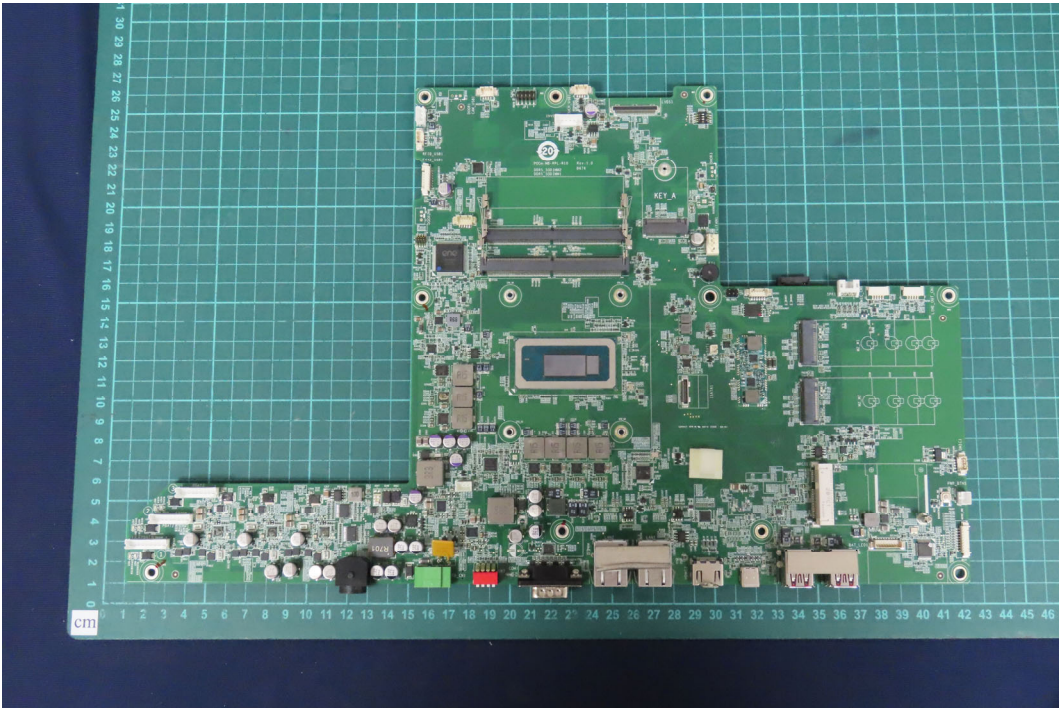
(153)EUT Photo
