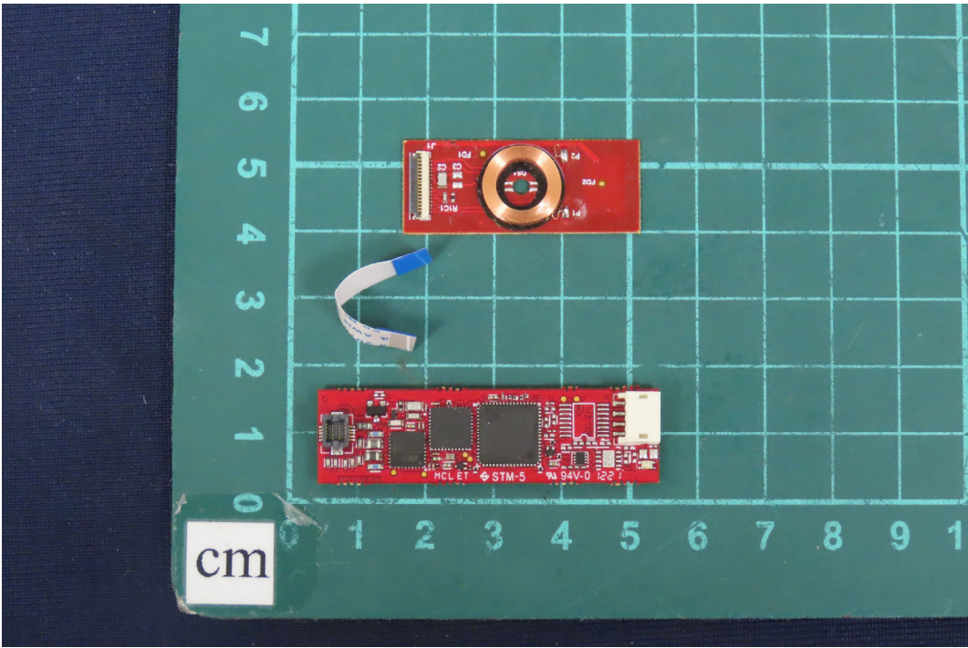
(160)EUT Photo
