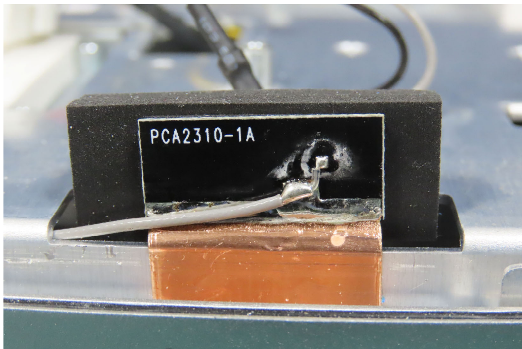
(48) EUT Photo
