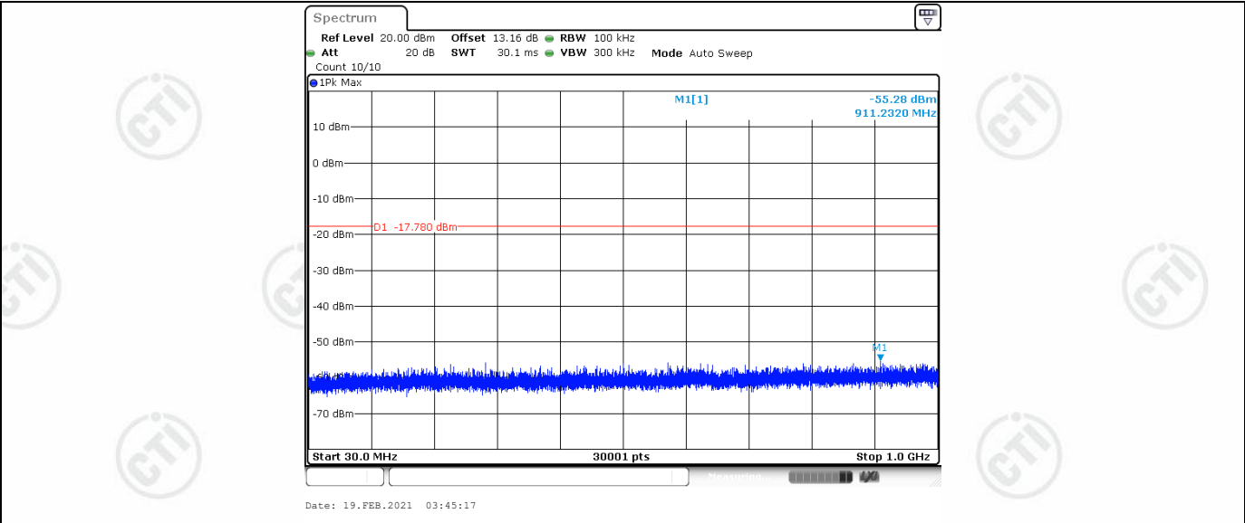
11G Ant2 2412 30~1000
