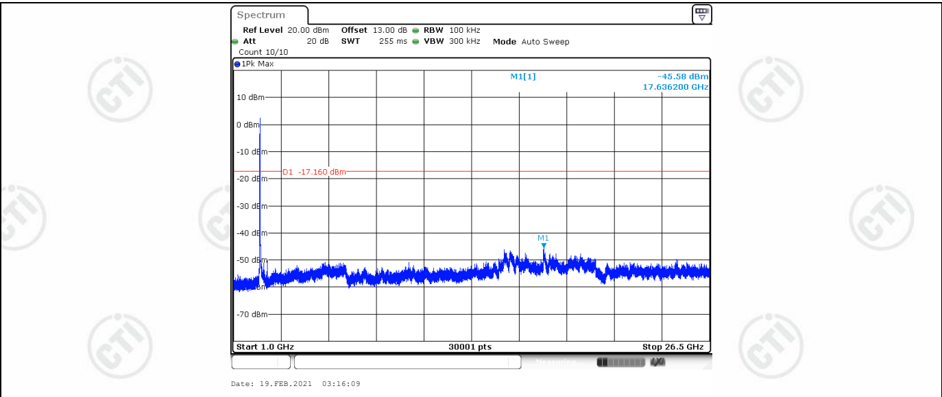
11G Ant1 2412 1000~26500
