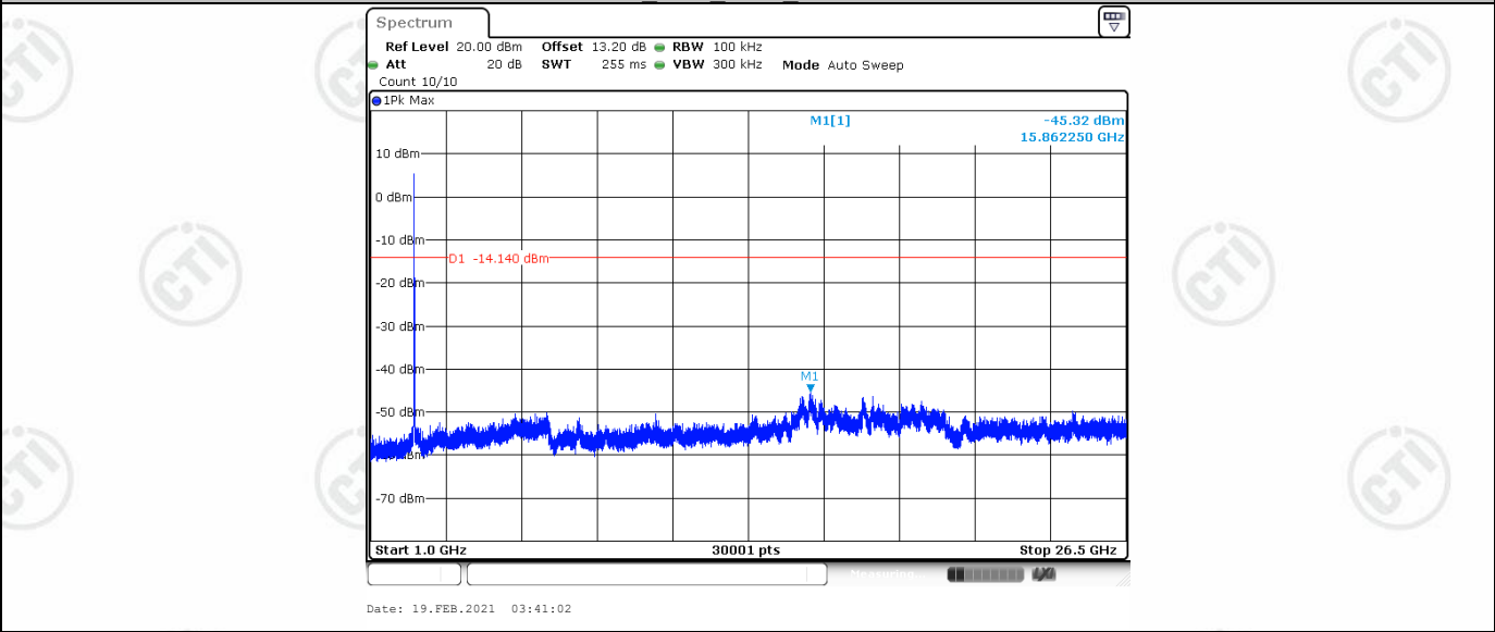
11B Ant2 2462 1000~26500
