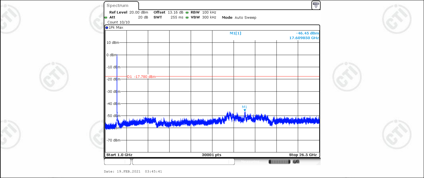
11G Ant2 2412 1000~26500
