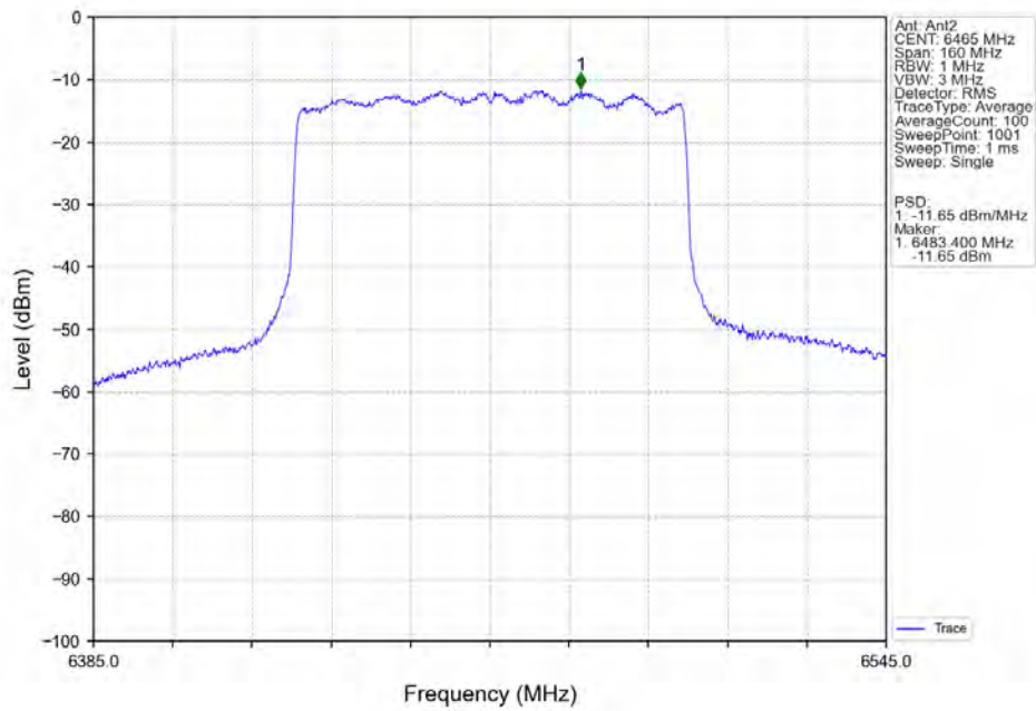
802.11ax(HEW80)_LCH_6465MHz_RU996_Left_MIMO_NTNV
