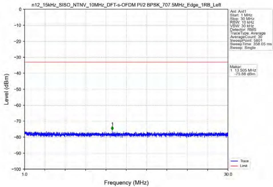
n12_15kHz_SISO_NTNV_10MHz_DFT-s-OFDM_PI/2_BPSK_707.5MHz_Edge_1RB_Left
