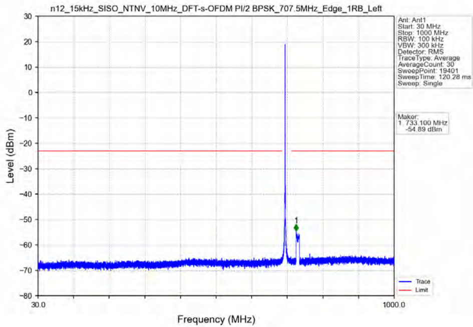
n12_15kHz_SISO_NTNV_10MHz_DFT-s-OFDM_PI/2_BPSK_707.5MHz_Edge_1RB_Left
