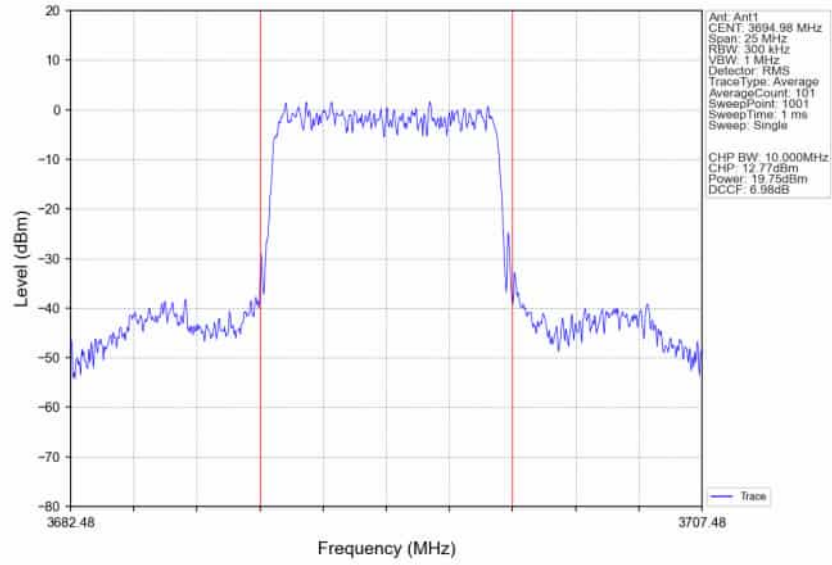
n48_30kHz_SISO_NTNV_10MHz_DFT-s-OFDM_PI/2_BPSK_3694.98MHz_Inner_Full
