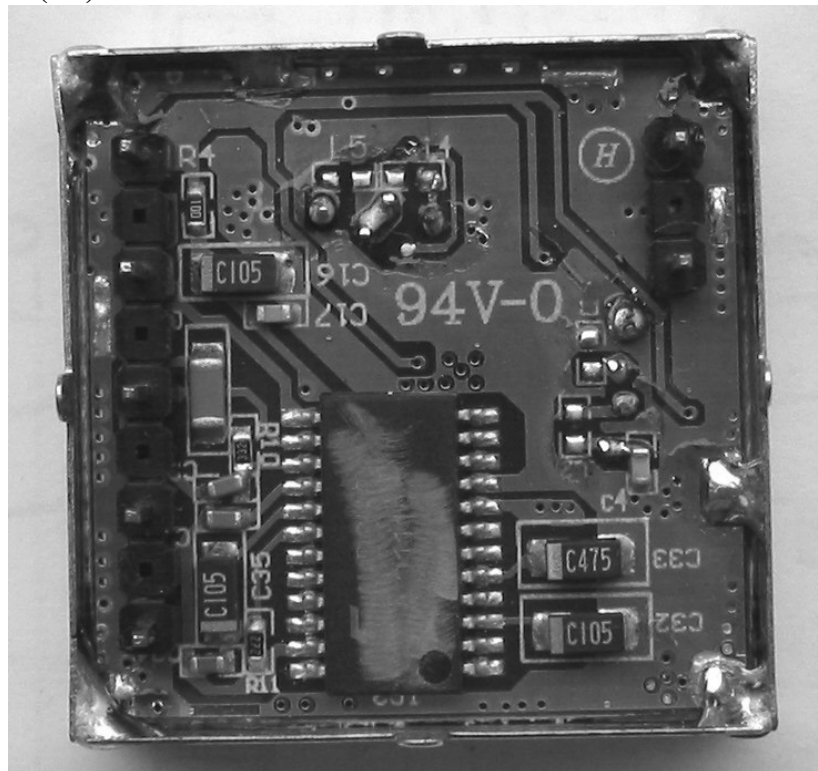
UHF module (Rx)
