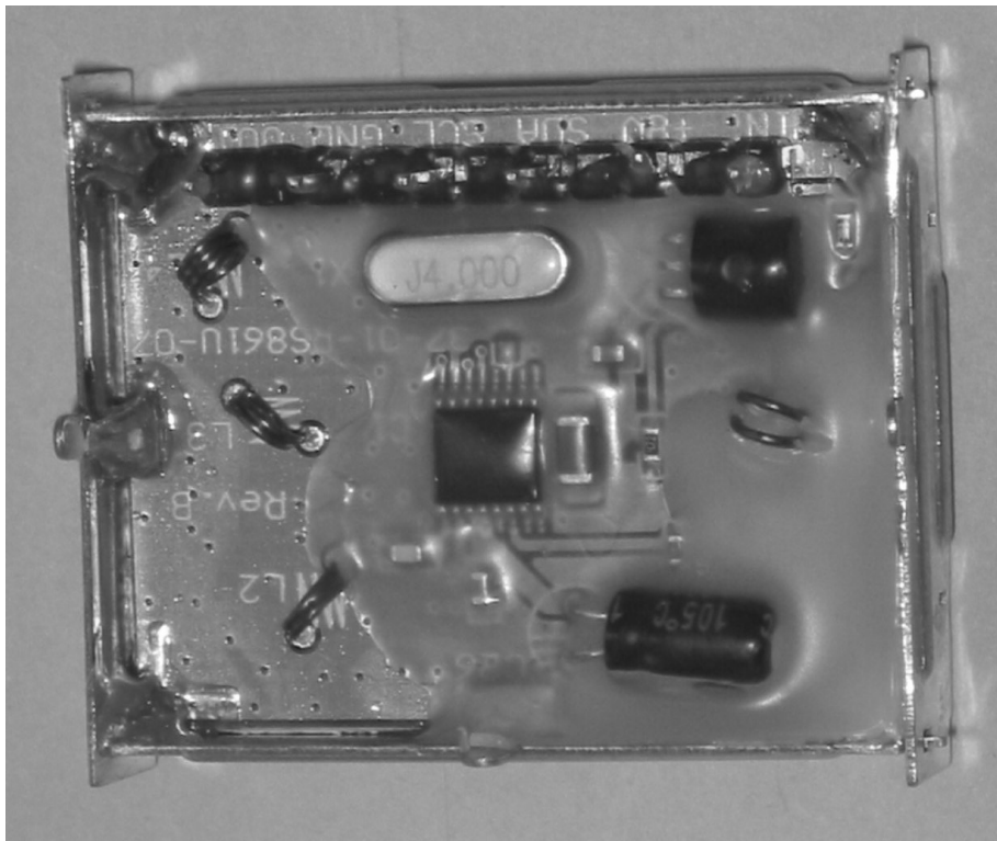
UHF module (Tx)
