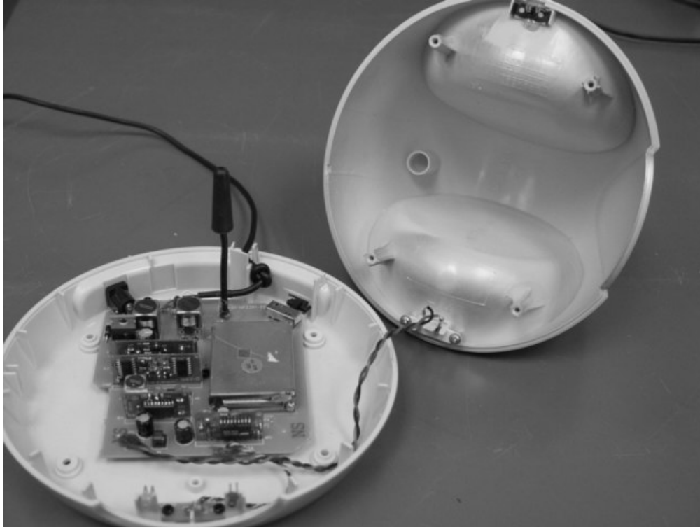
HP2791, HP2391, HP2491, HP2691, HP2891 and HP1991 internal photo
