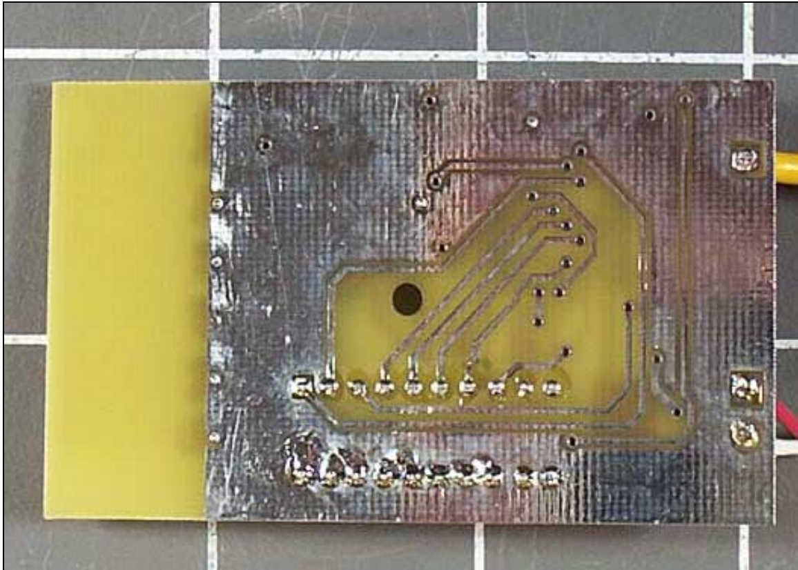
PCB Bottom
