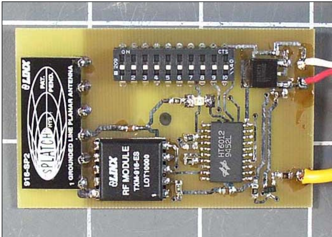
PCB Top
