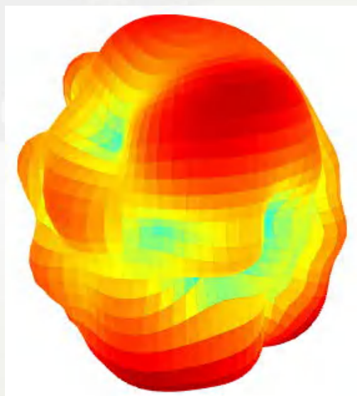
5180MHz
