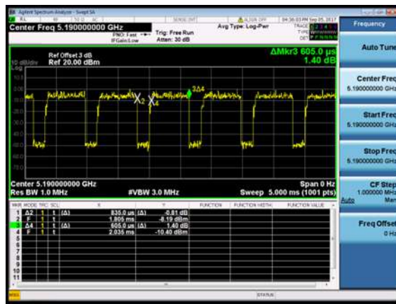
802.11ac(40MHz) 5190MHz
