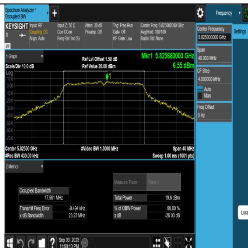
11N20ISO-Ant1-5825
