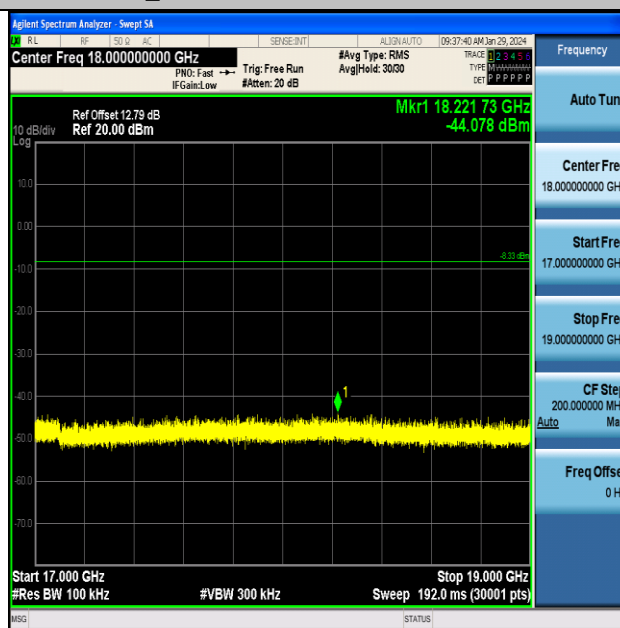
BLE_2M-Ant1-2402-17000~19000-PASS
