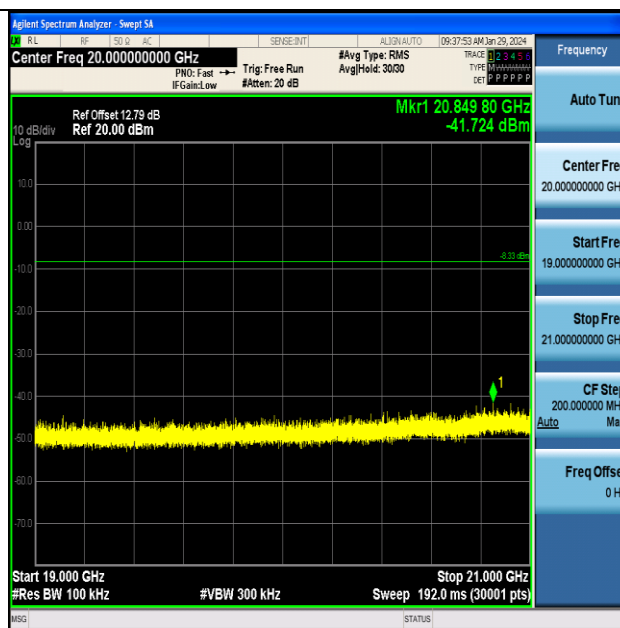
BLE_2M-Ant1-2402-19000~21000-PASS
