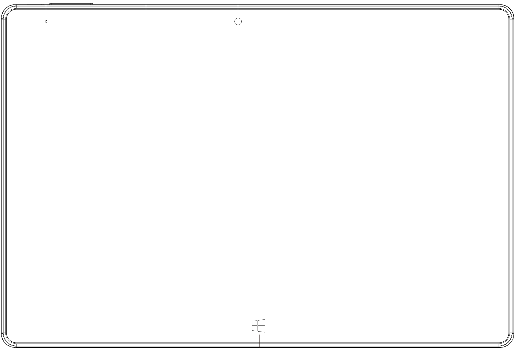
Windows图标
