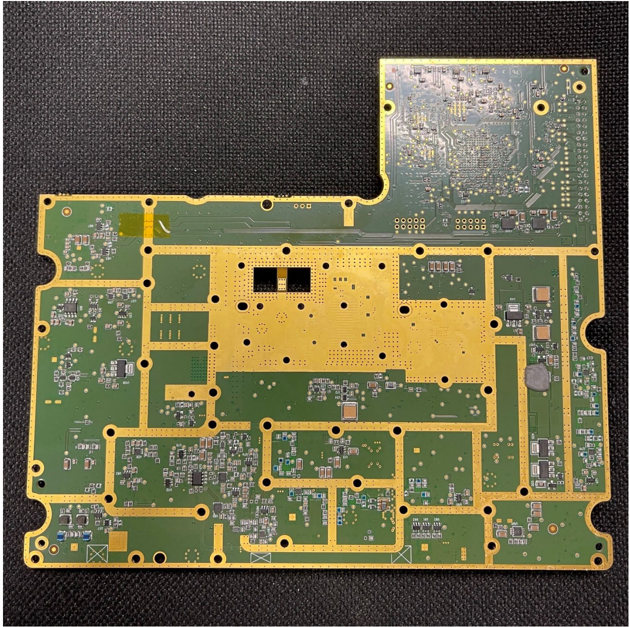
RF PCBA - TOP
