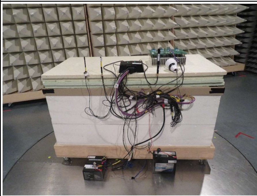
EUT setup
