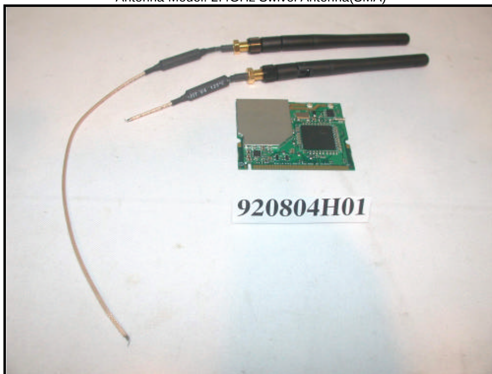
Antenna Model: 2.4GHz Swivel Antenna(SMA)
