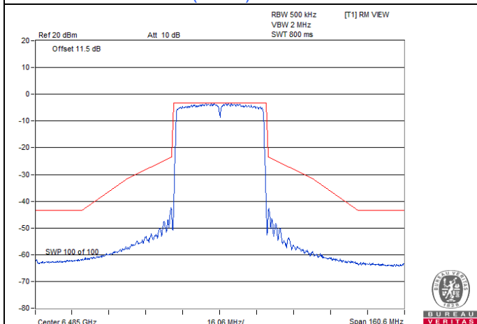
802.11ax (HE40) / Chain 3 : CH 107
