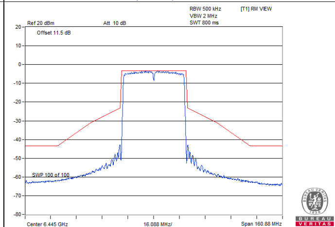
802.11ax (HE40) / Chain 3 : CH 99
