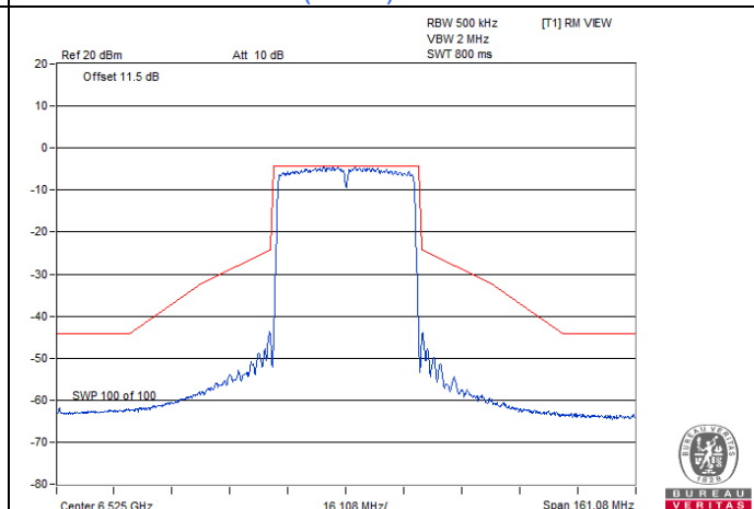
802.11ax (HE40) / Chain 3 : CH 115
