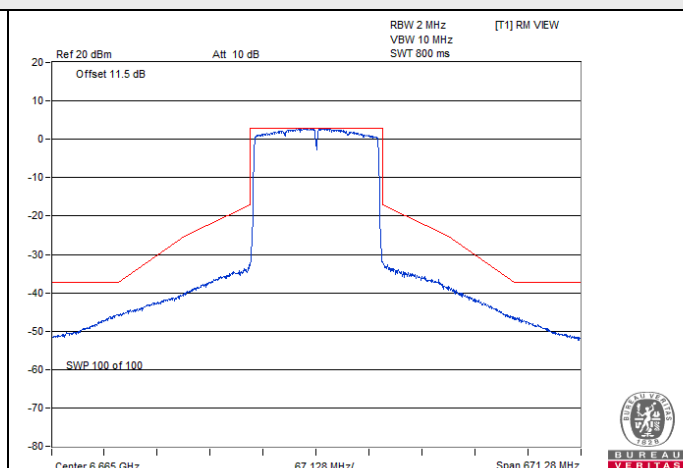
802.11ax (HE160) / Chain 3 : CH 143
