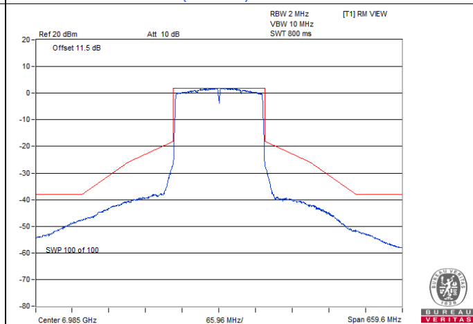
802.11ax (HE160) / Chain 3 : CH 207
