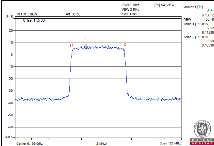
802.11ax (HE40) Beamforming / Chain 0 : CH 43
