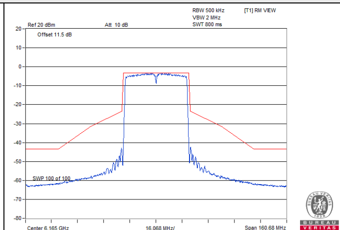
802.11ax (HE40) / Chain 3 : CH 43
