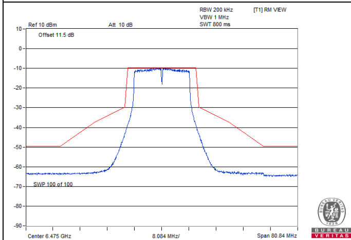
802.11a / Chain 2 : CH 105
