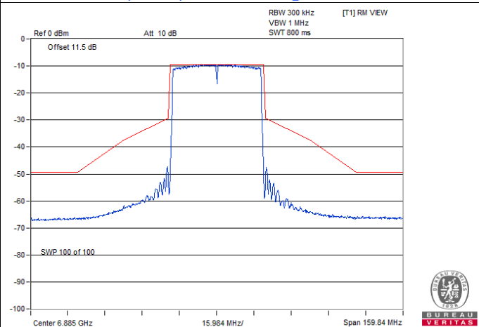
802.11ax (HE40) Beamforming / Chain 0 : CH 187
