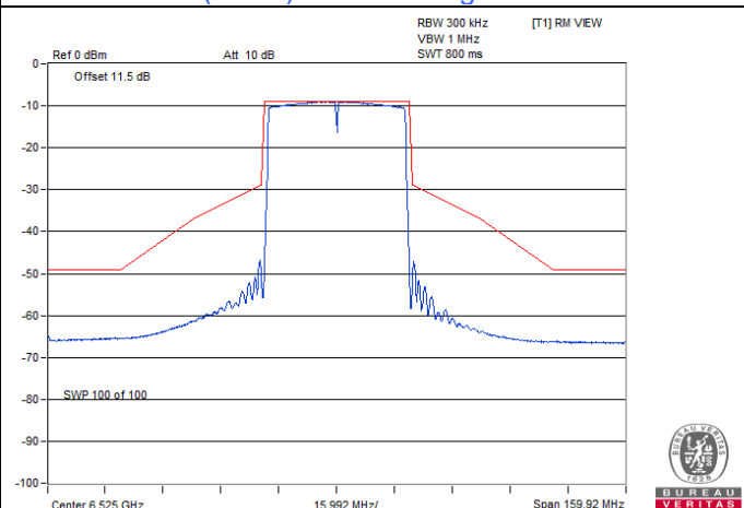
802.11ax (HE40) Beamforming / Chain 1 : CH 115
