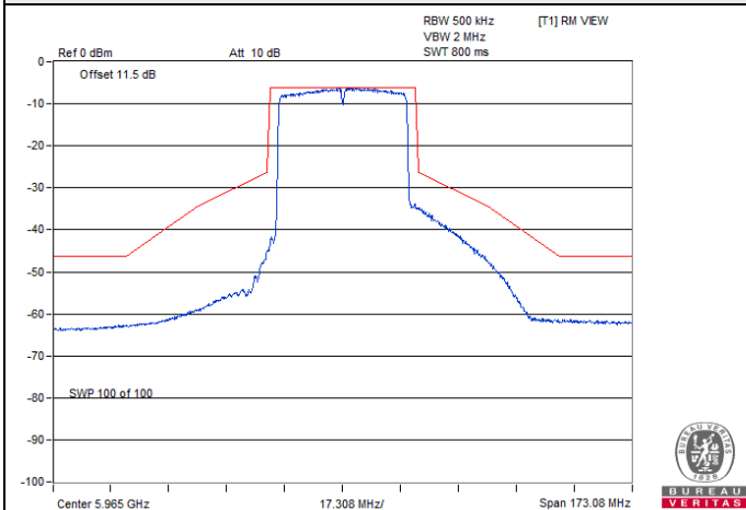
802.11ax (HE40) Beamforming / Chain 3 : CH 3
