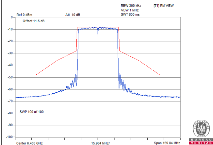
802.11ax (HE40) Beamforming / Chain 3 : CH 91
