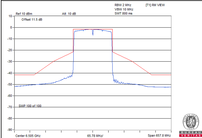
802.11ax (HE160) Beamforming / Chain 1 : CH 111
