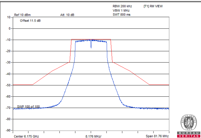
802.11a / Chain 2 : CH 45
