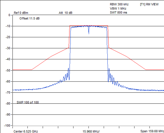
802.11ax (HE40) Beamforming / Chain 2 : CH 115
