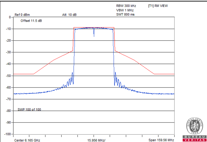
802.11ax (HE40) Beamforming / Chain 3 : CH 43
