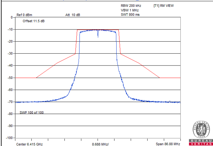
802.11ax (HE20) Beamforming / Chain 3 : CH 93
