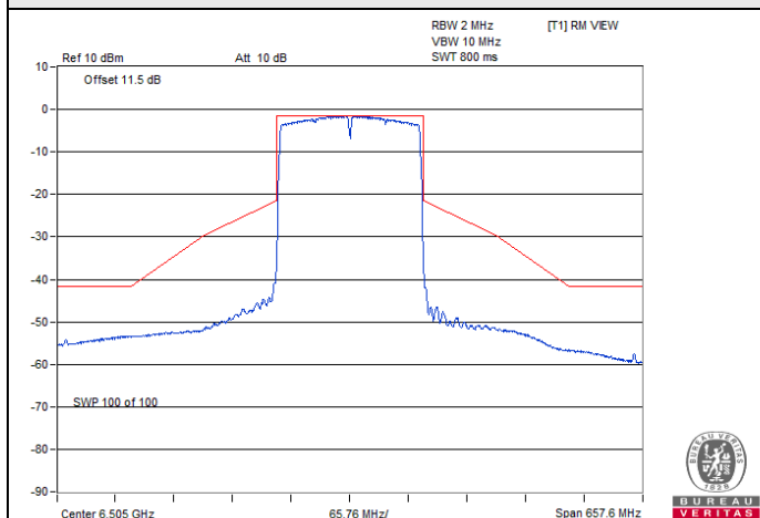
802.11ax (HE160) Beamforming / Chain 3 : CH 111
