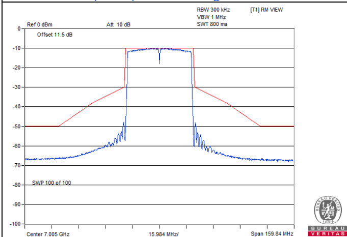
802.11ax (HE40) Beamforming / Chain 1 : CH 211
