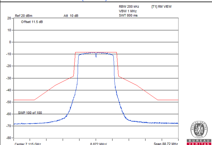
802.11ax (HE20) / Chain 3 : CH 233
