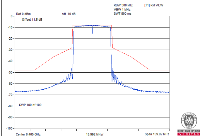
802.11ax (HE40) Beamforming / Chain 1 : CH 91
