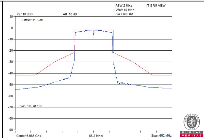
802.11ax (HE160) Beamforming / Chain 1 : CH 207
