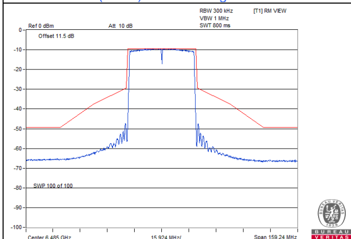
802.11ax (HE40) Beamforming / Chain 1 : CH 107
