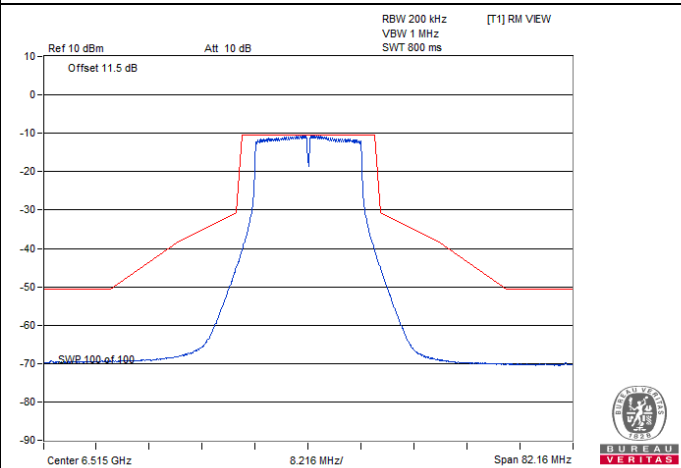
802.11a / Chain 2 : CH 113
