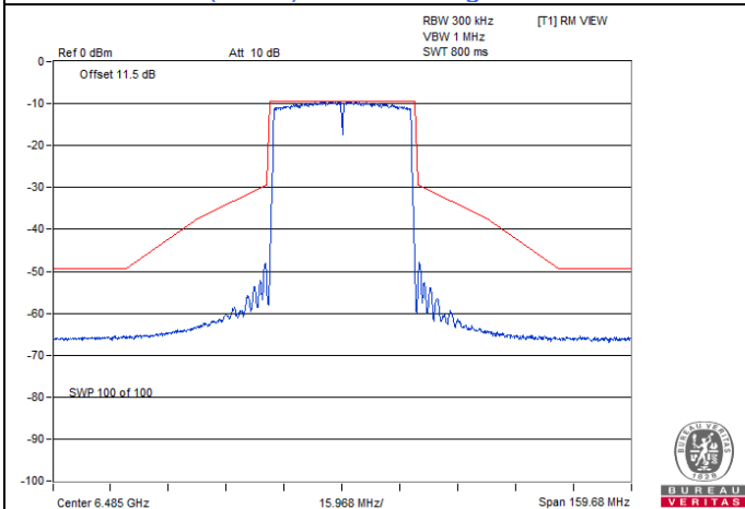
802.11ax (HE40) Beamforming / Chain 3 : CH 107
