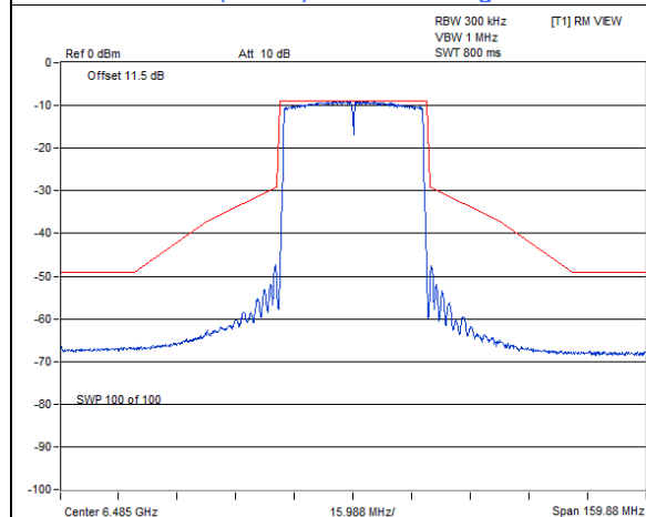
802.11ax (HE40) Beamforming / Chain 0 : CH 107
