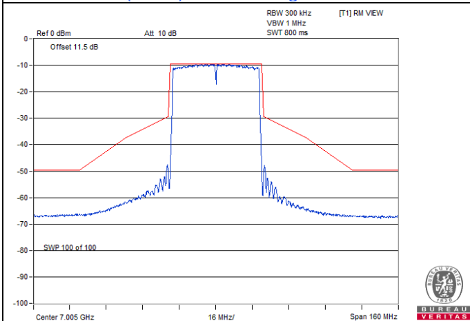
802.11ax (HE40) Beamforming / Chain 0 : CH 211
