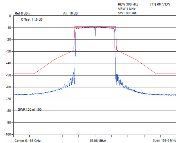
802.11ax (HE40) Beamforming / Chain 2 : CH 43
