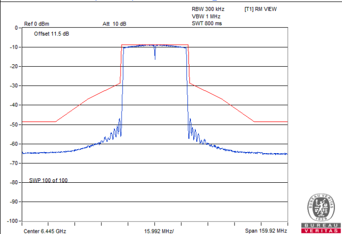
802.11ax (HE40) Beamforming / Chain 1 : CH 99
