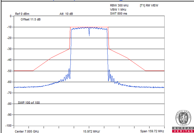
802.11ax (HE40) Beamforming / Chain 3 : CH 211
