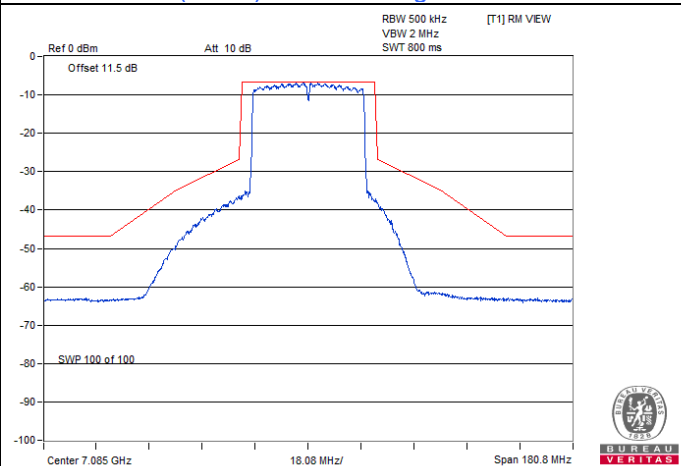
802.11ax (HE40) Beamforming / Chain 3 : CH 227
