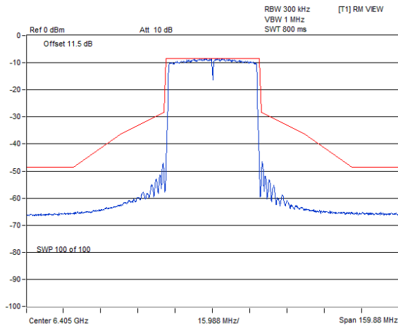
802.11ax (HE40) Beamforming / Chain 2 : CH 91
