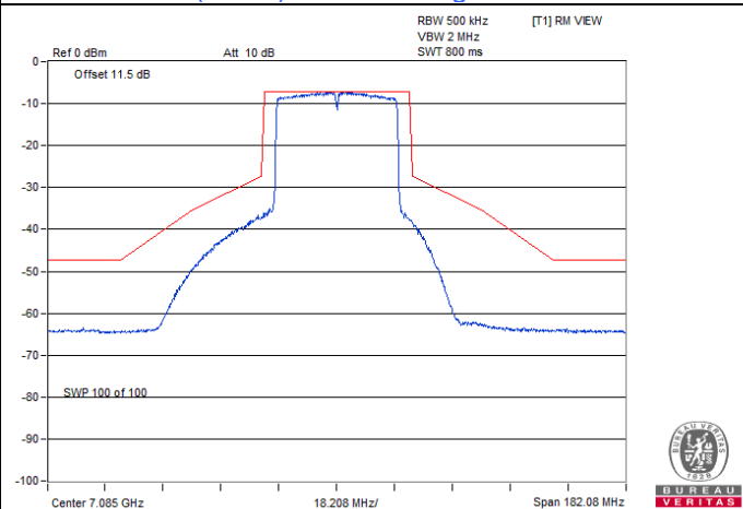
802.11ax (HE40) Beamforming / Chain 1 : CH 227
