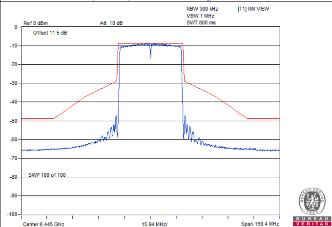
802.11ax (HE40) Beamforming / Chain 3 : CH 99
