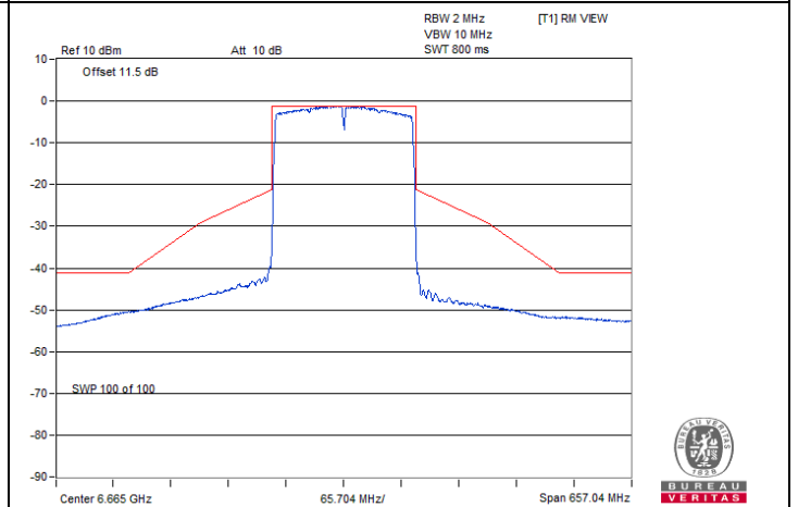
802.11ax (HE160) Beamforming / Chain 1 : CH 143
