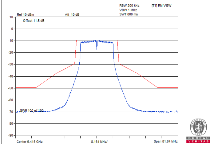
802.11a / Chain 2 : CH 93
