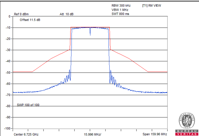
802.11ax (HE40) Beamforming / Chain 0 : CH 155
