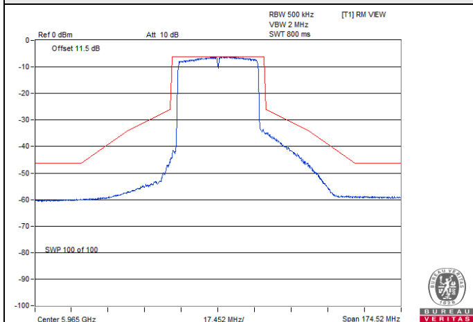
802.11ax (HE40) Beamforming / Chain 1 : CH 3
