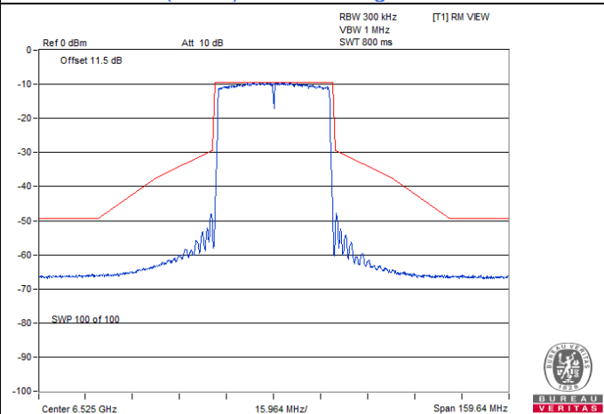
802.11ax (HE40) Beamforming / Chain 3 : CH 115
