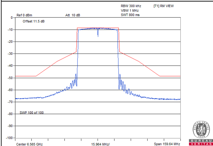
802.11ax (HE40) Beamforming / Chain 0 : CH 123
