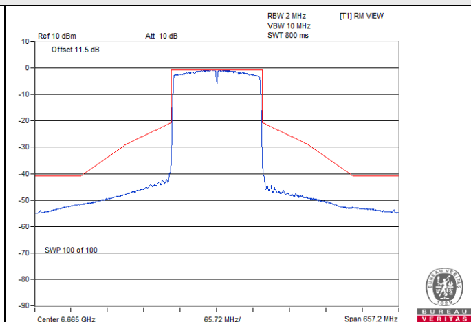
802.11ax (HE160) Beamforming / Chain 3 : CH 143
