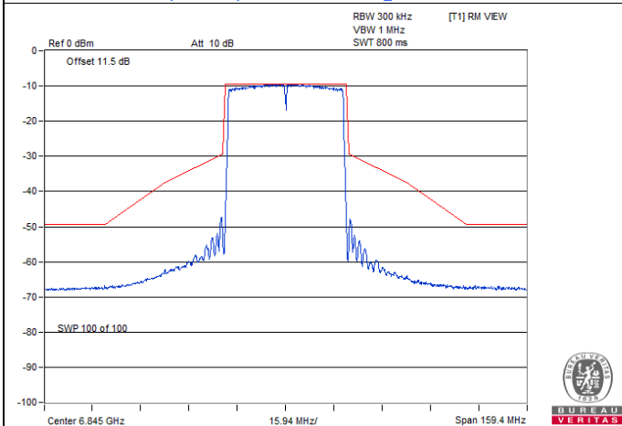
802.11ax (HE40) Beamforming / Chain 0 : CH 179
