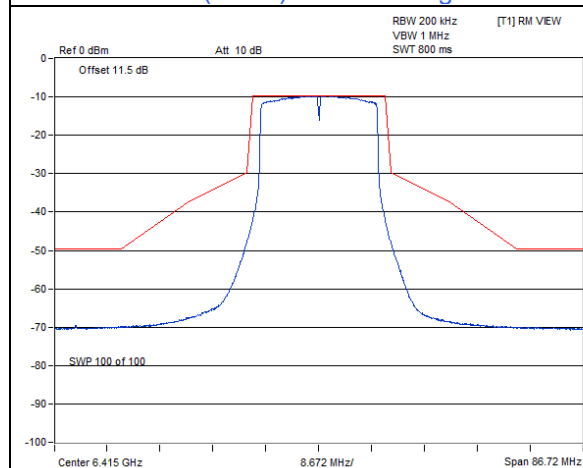
802.11ax (HE20) Beamforming / Chain 0 : CH 93
