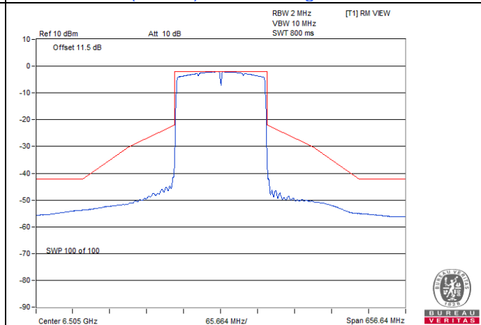
802.11ax (HE160) Beamforming / Chain 2 : CH 111
