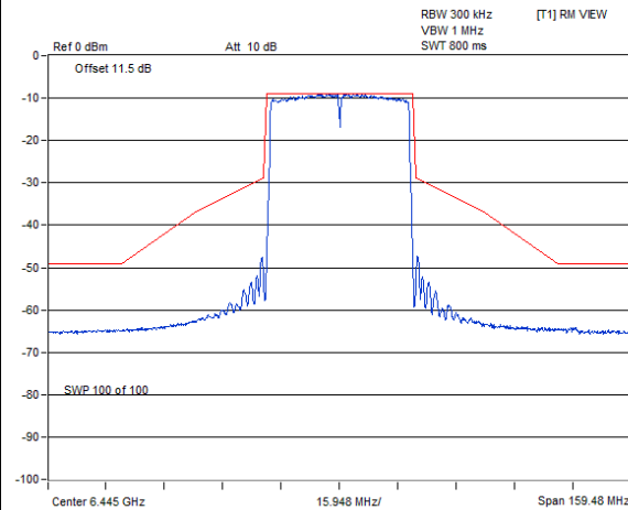
802.11ax (HE40) Beamforming / Chain 2 : CH 99
