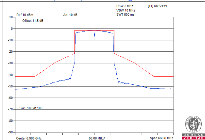
802.11ax (HE160) Beamforming / Chain 3 : CH 207
