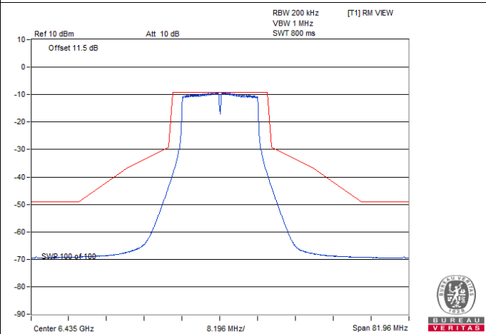
802.11a / Chain 2 : CH 97
