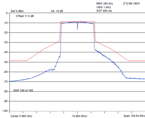
802.11ax (HE40) Beamforming / Chain 2 : CH 3
