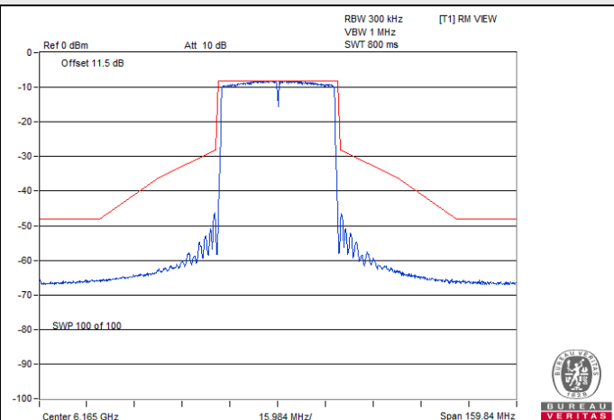
802.11ax (HE40) Beamforming / Chain 1 : CH 43
