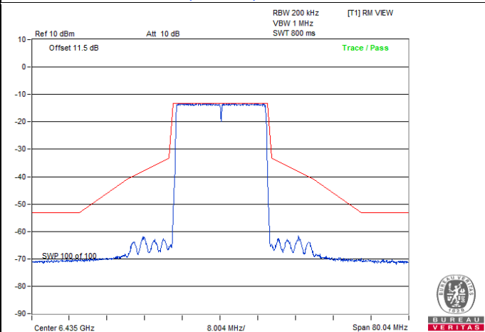
802.11be (EHT20) / Chain 3 : CH 97
