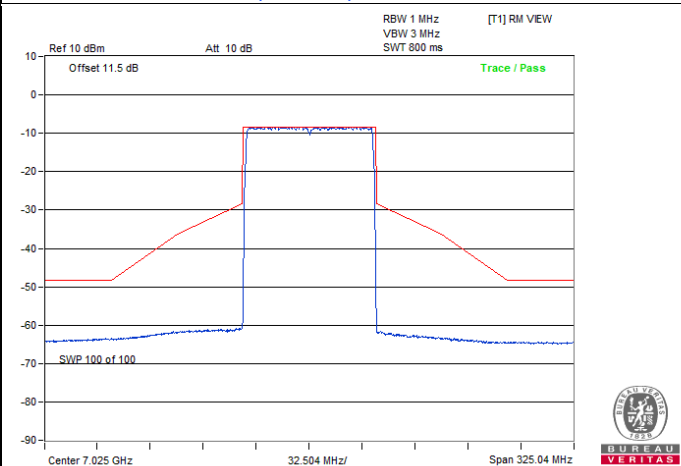
802.11be (EHT80) / Chain 3 : CH 215
