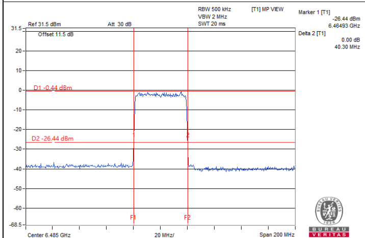
802.11be (EHT40) / Chain 3 : CH 107
