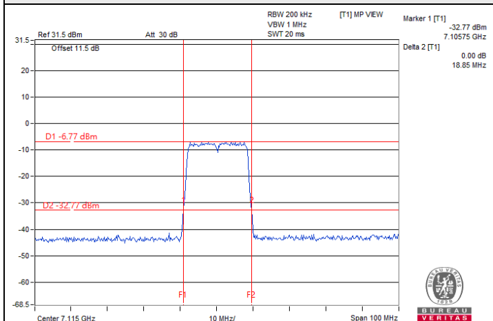
802.11a / Chain 2 : CH 233
