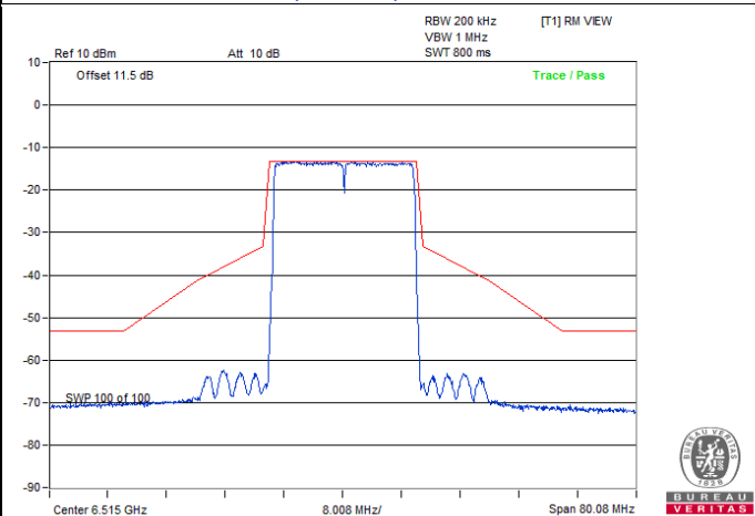
802.11be (EHT20) / Chain 3 : CH 113
