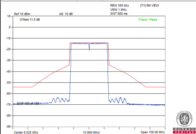
802.11be (EHT40) / Chain 2 : CH 115
