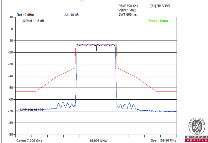
802.11be (EHT40) / Chain 1 : CH 211
