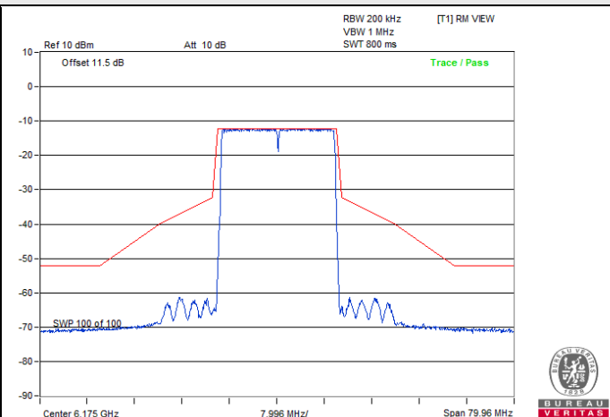
802.11be (EHT20) / Chain 3 : CH 45
