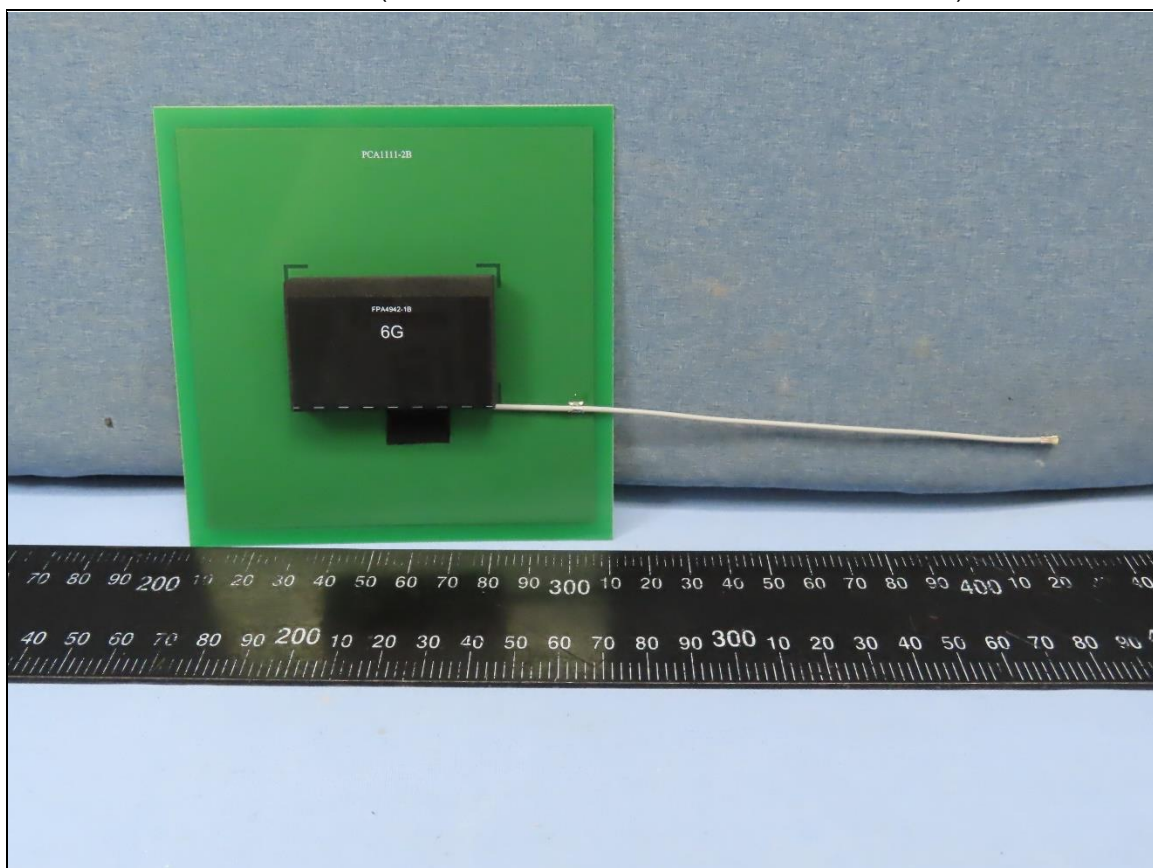
Antenna Set 4 (Brand: INPAQ / Model: RFFPA494217EM6B901)
