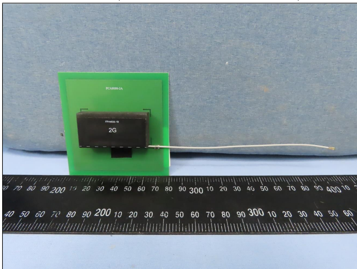
Antenna Set 2 (Brand: INPAQ / Model: RFFPA493517EMAB901)
