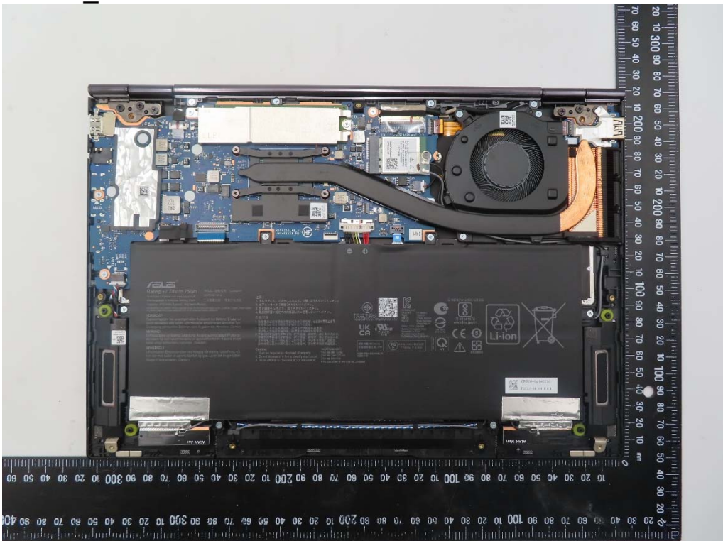
Internal_Antenna_INPAQ
