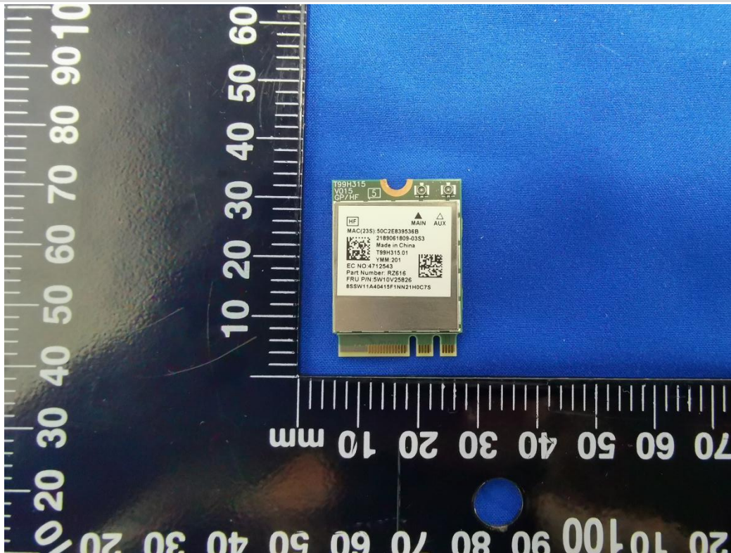
RF MODULE TOP VIEW_MT7922A22M
