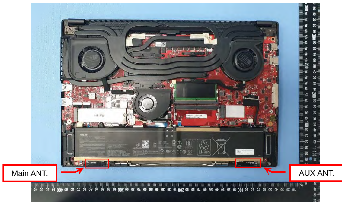
EUT Photo (2)
