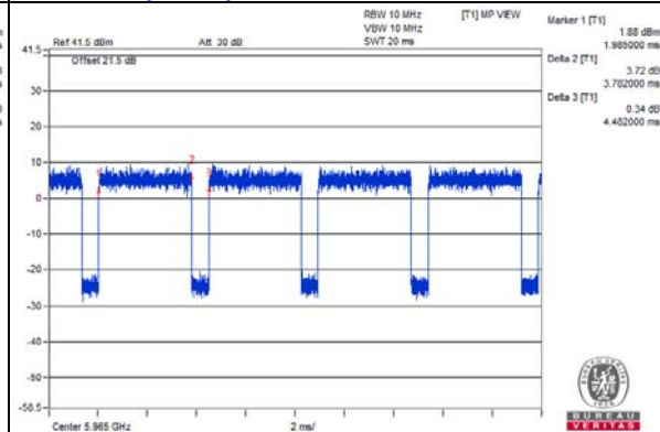
802.11ax (HE40)
