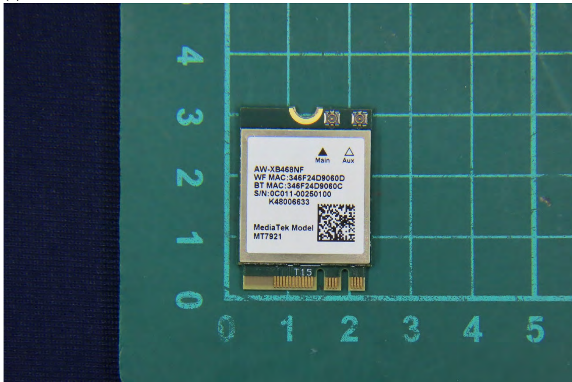
(4) EUT Photo
