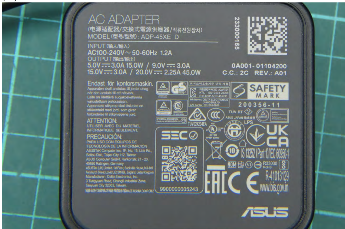
(30) EUT Photo
