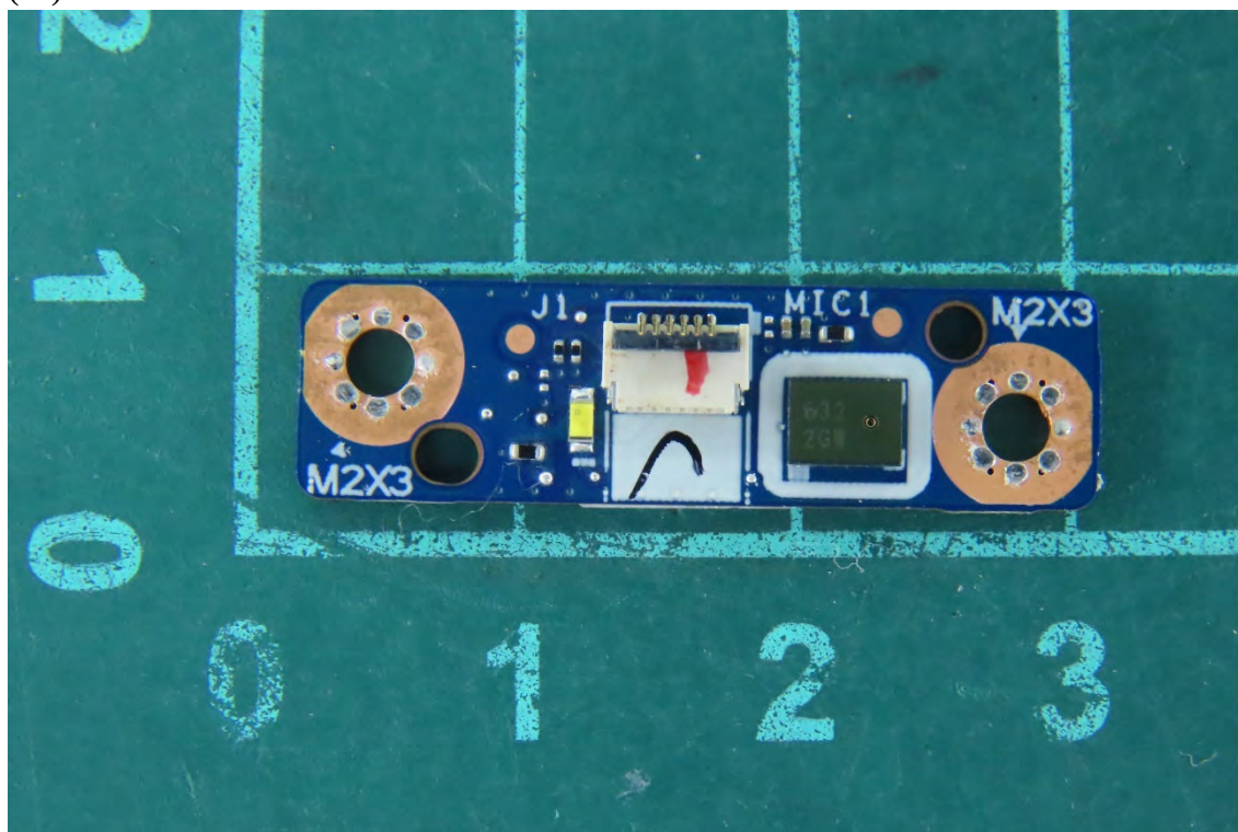
(15) EUT Photo
