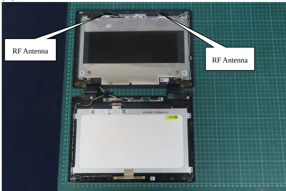
(24) EUT Photo
