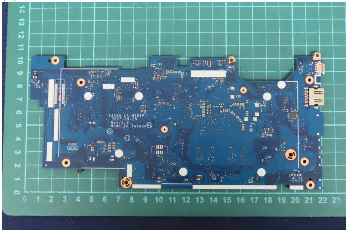
(20) EUT Photo
