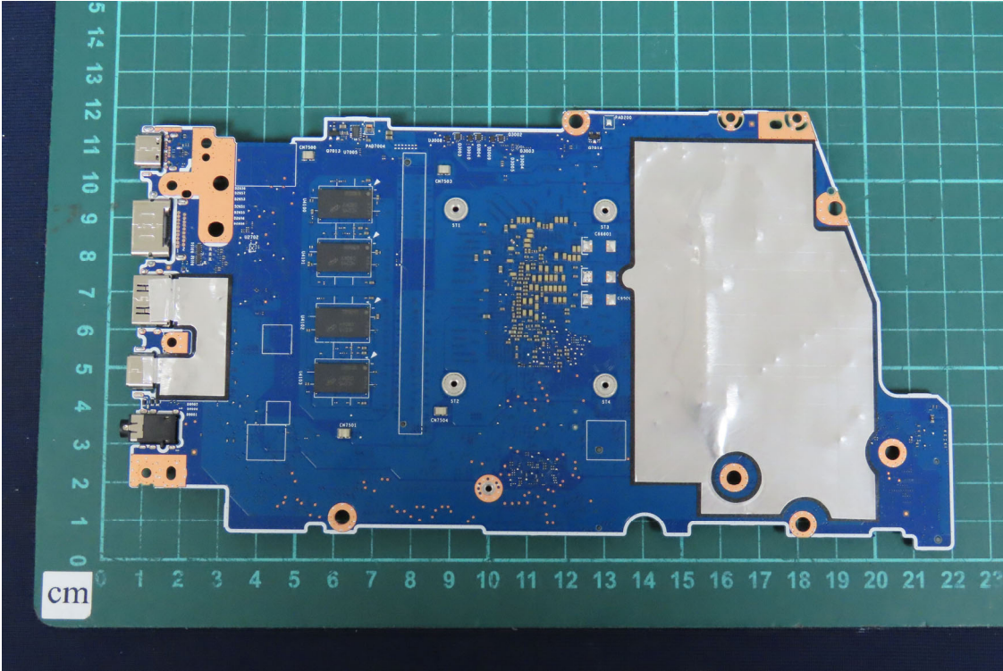
(36) EUT Photo
