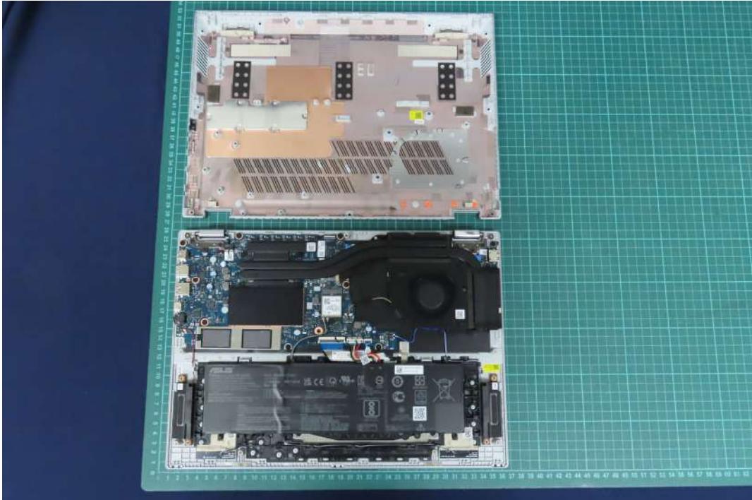
(9) EUT Photo
