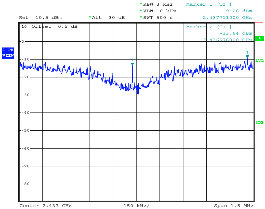
Plot: B3B1 (1Mbps)
