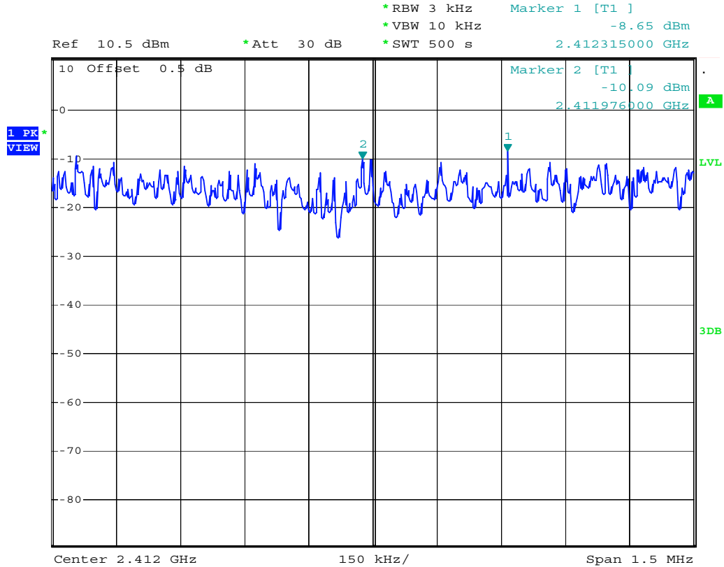
Plot: B3A1 (1Mbps)
