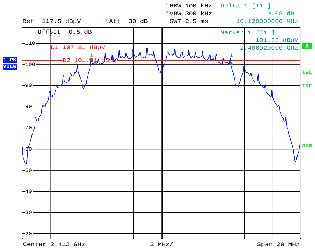
Plot: B2A1 (1Mbps)
