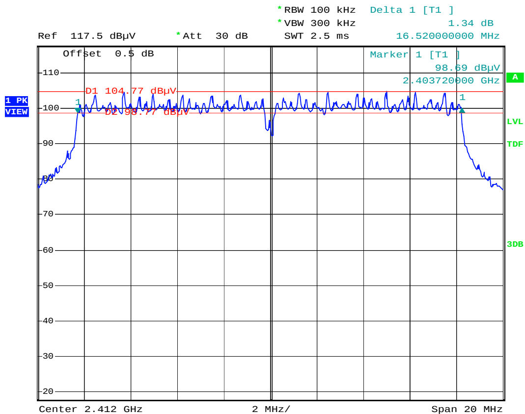
Plot: G2A2 (54Mbps)
