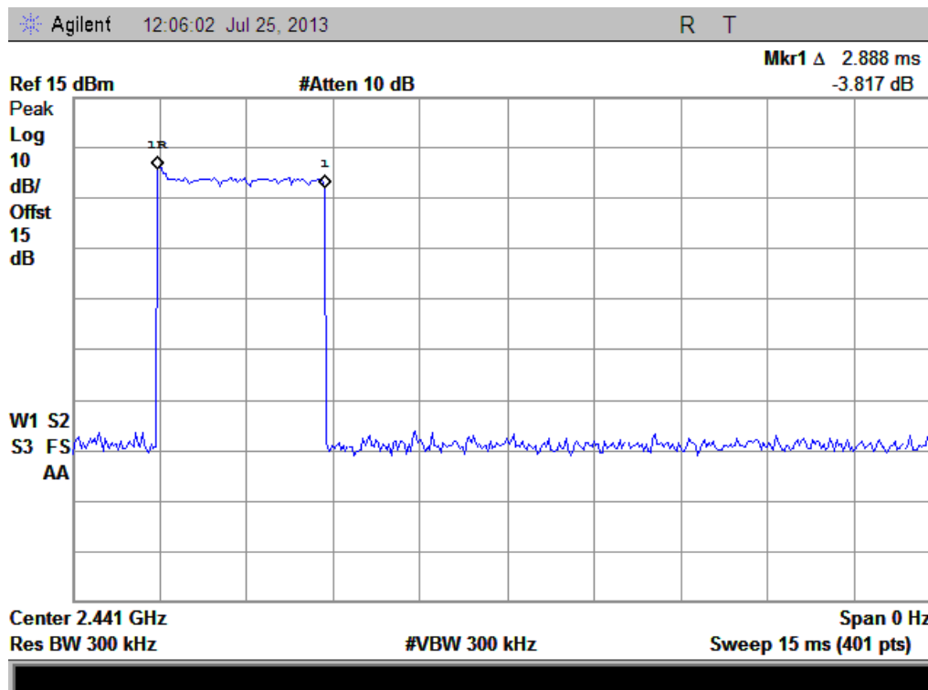
(Plot A: 1DH5 @ GFSK)
