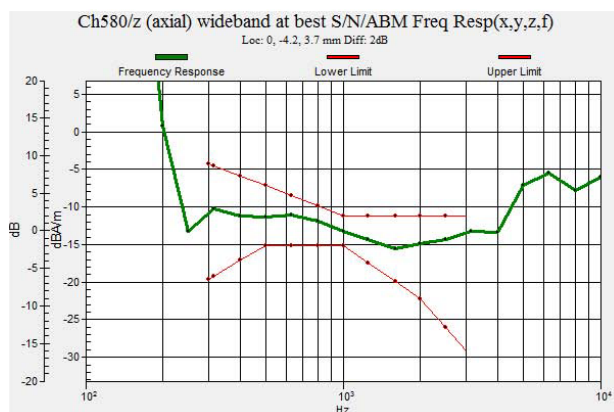
Fig 7.3 CDMA2000 BC10 Ch580
