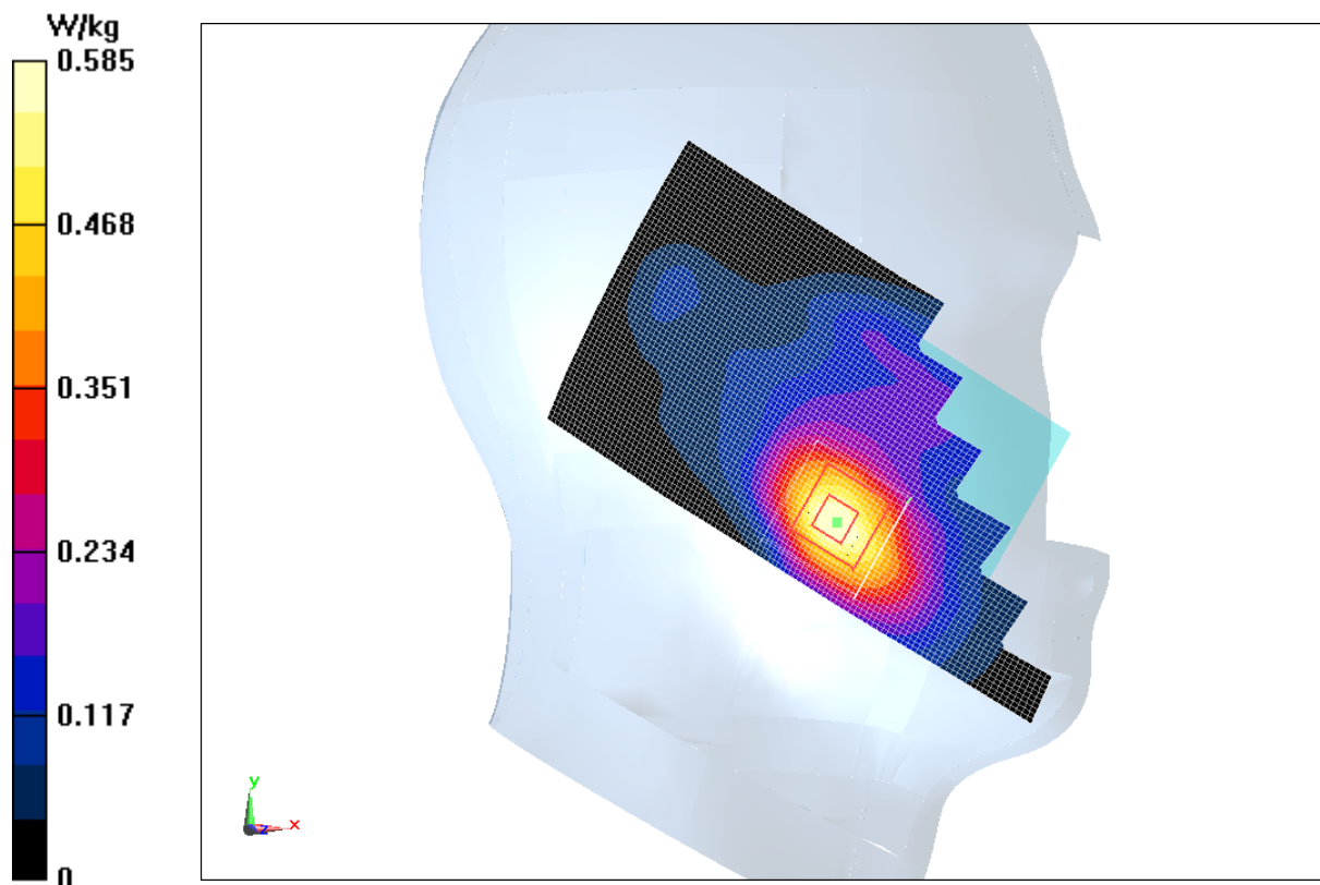
Fig.7 WCDMA1900 CH9262
