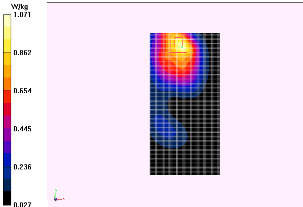
Fig.8 WCDMA1900 CH9400
