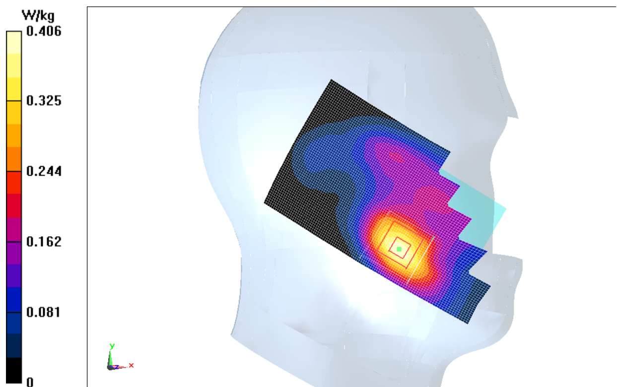
Fig.7 WCDMA1700 CH1412
