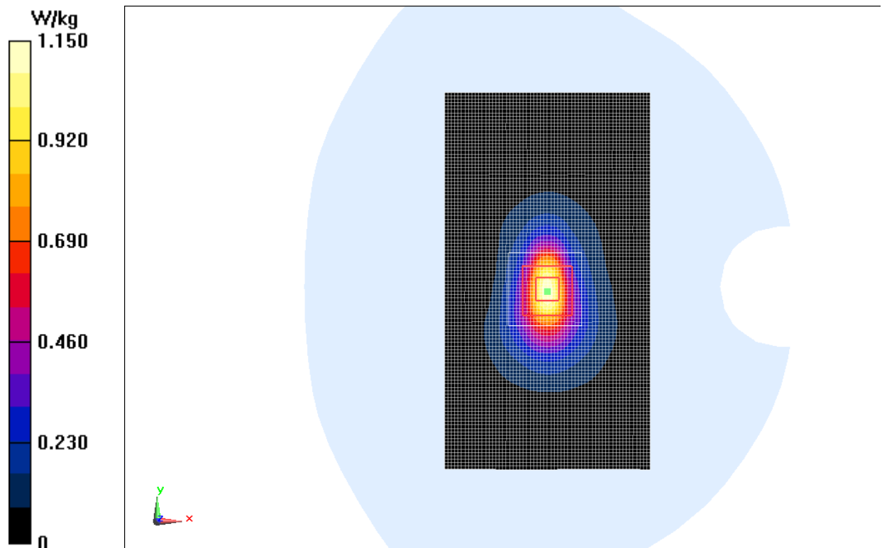
Fig.8 WCDMA1700 CH1412
