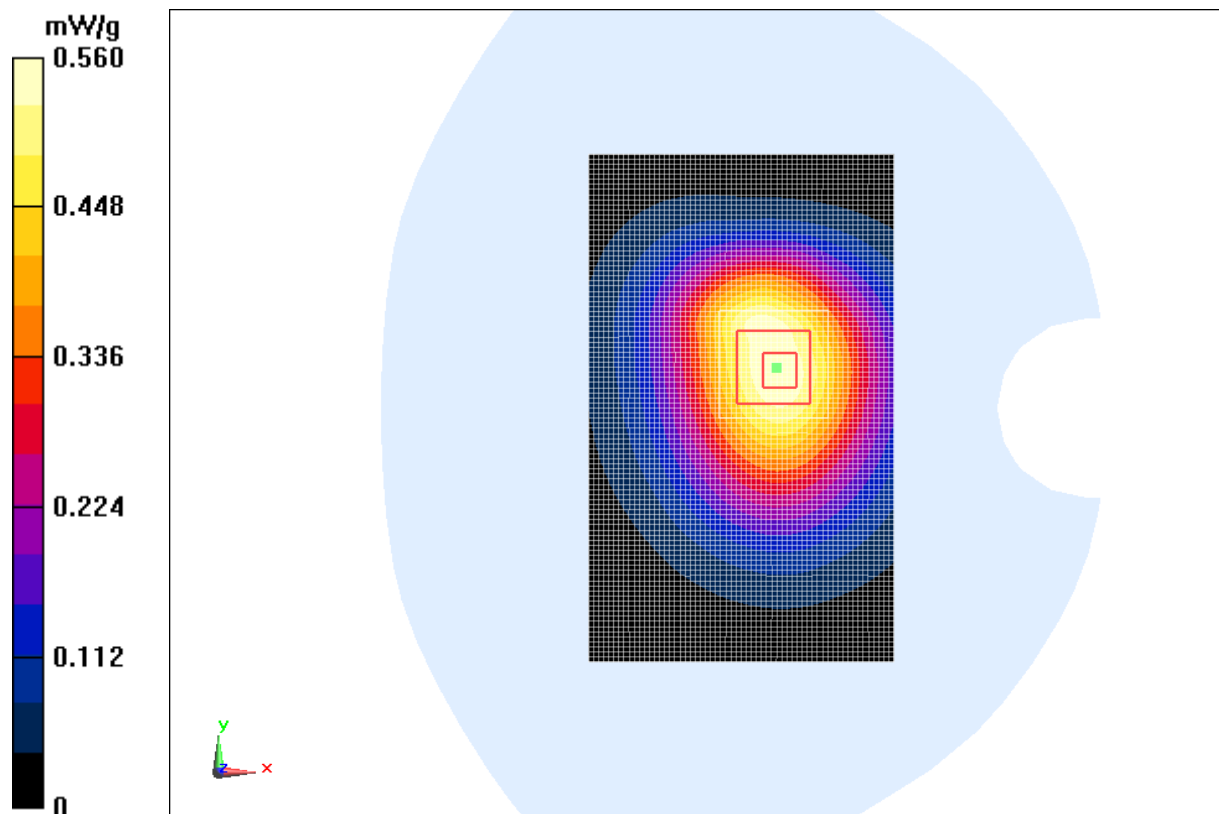
Fig. 23 850 MHz CH190
