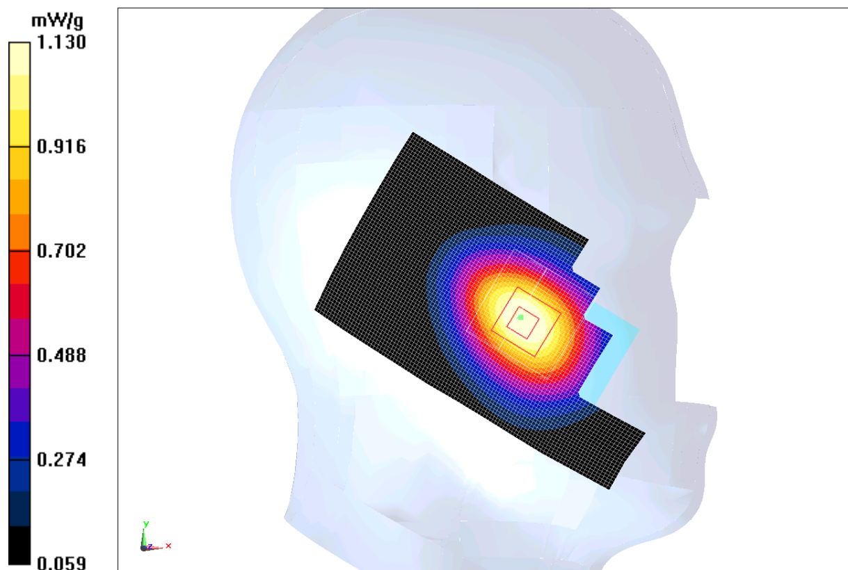
Fig. 1 850MHz CH251
