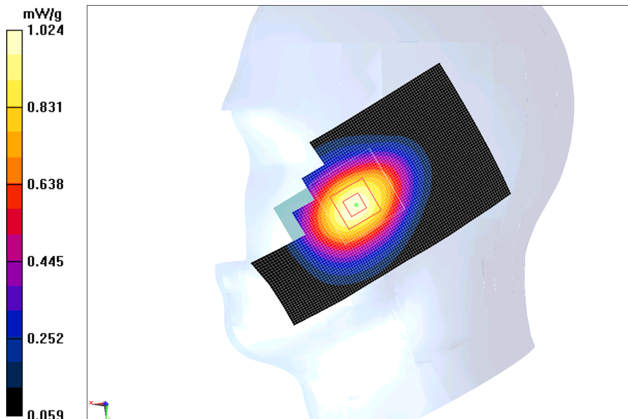
Fig. 8 850 MHz CH190
