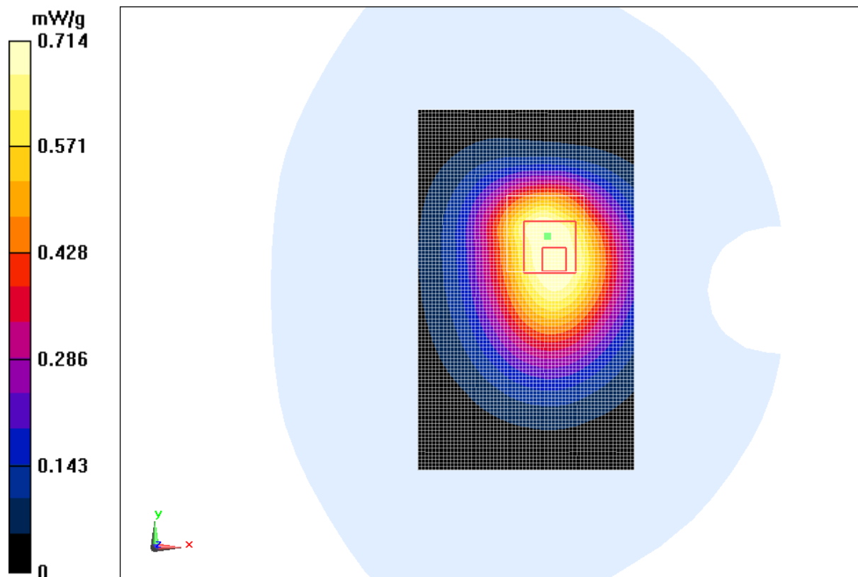
Fig. 21 850 MHz CH190
