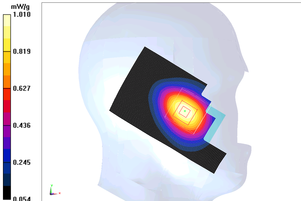
Fig. 2 850 MHz CH190
