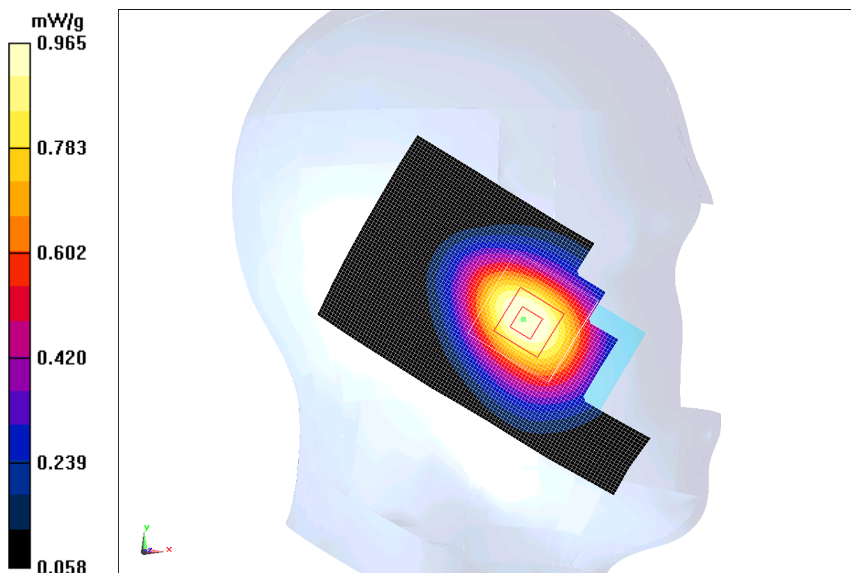
Fig. 15 850MHz CH251
