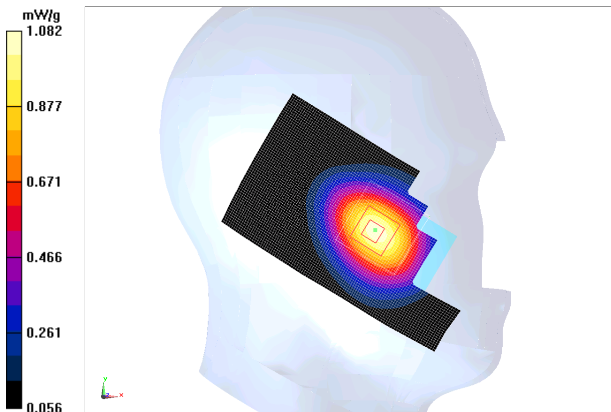
Fig. 16 850MHz CH251
