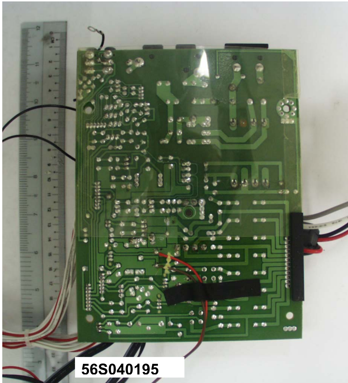
AV Unit – Power Supply Trace Side
