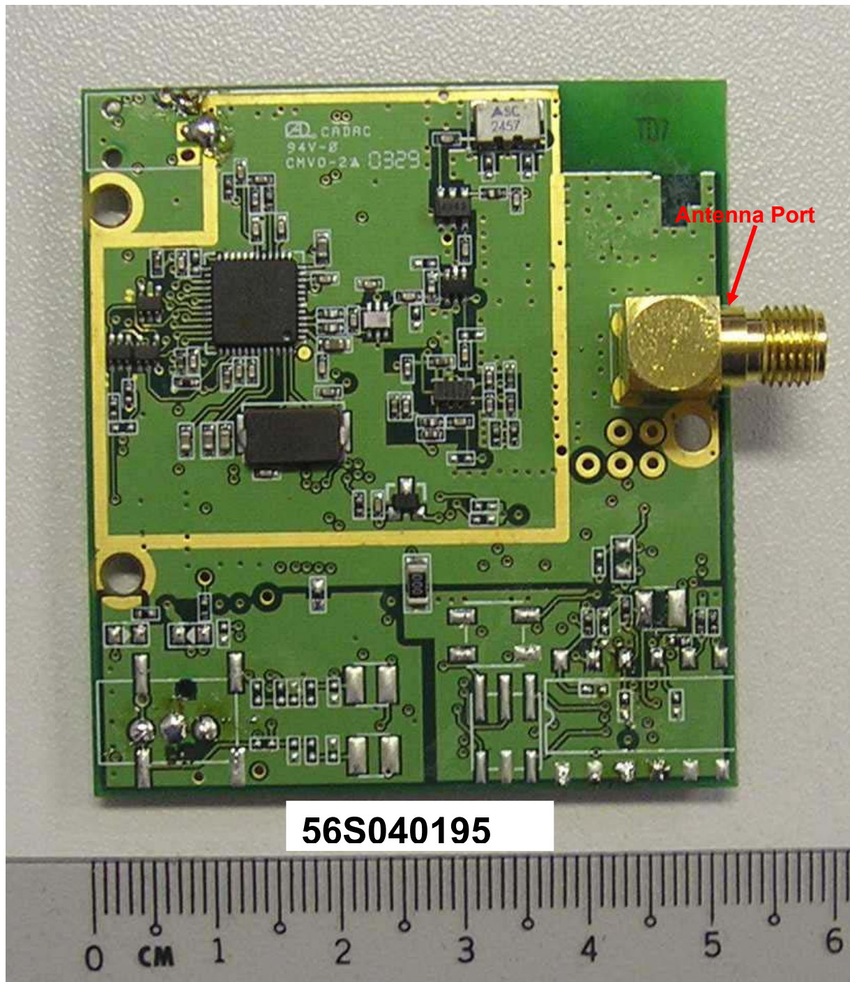
AV Unit – RF Board Trace Side
