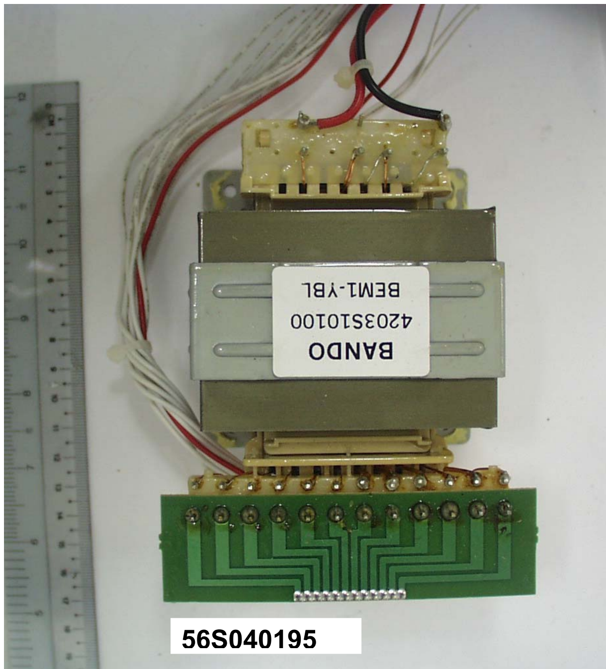
AV Unit – Power Transformer Board Component View 1
