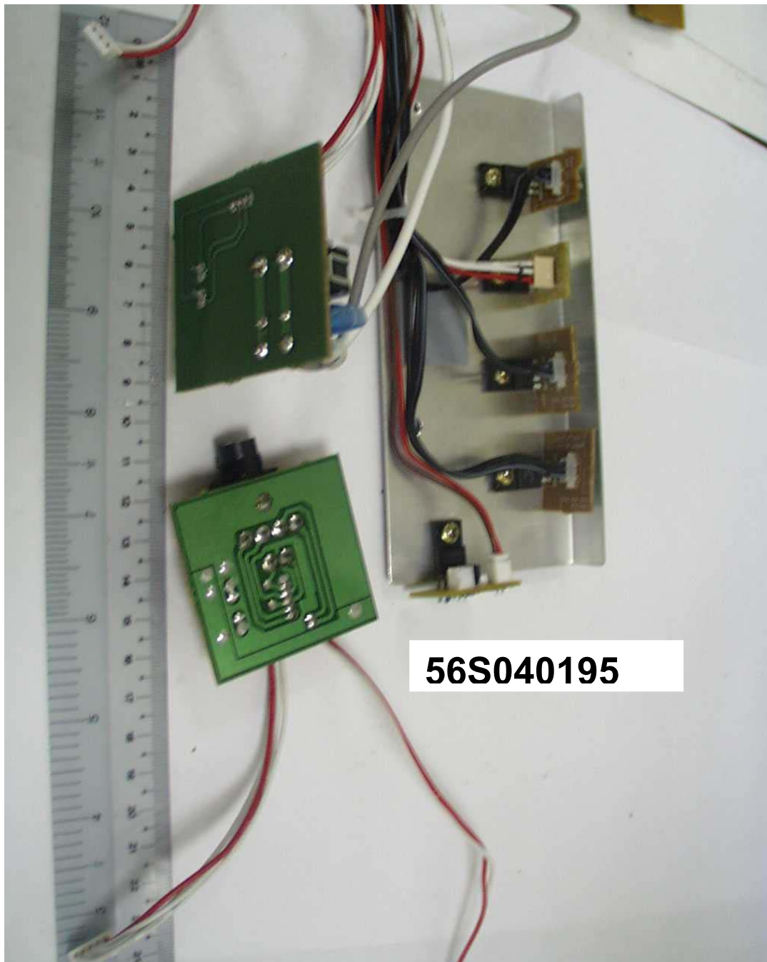
AV Unit – Power Supply Sub-Board Trace Side
