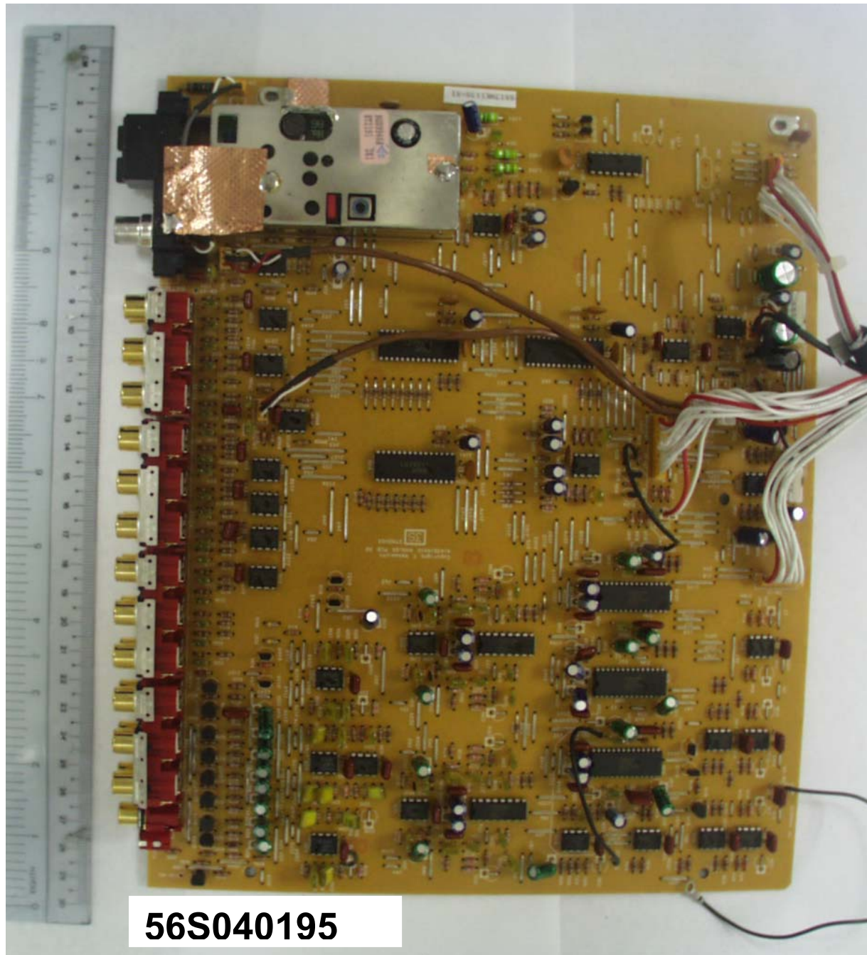
AV Unit – Analog Component Side
