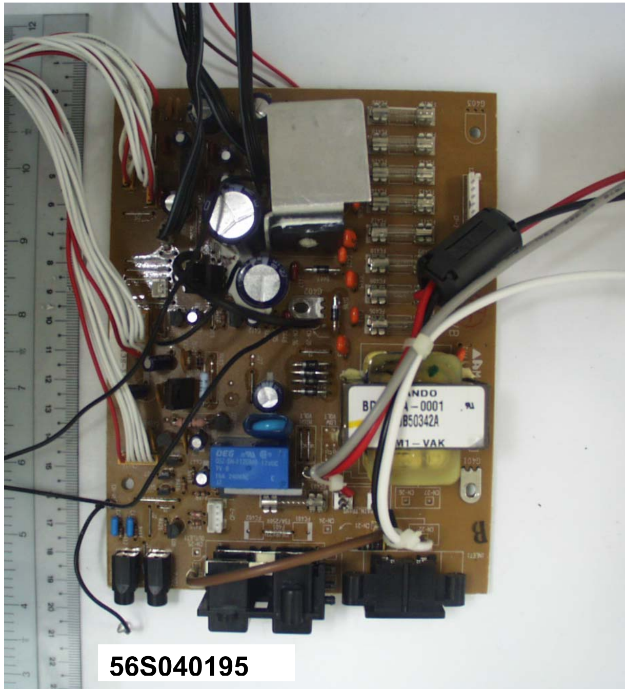
AV Unit – Power Supply Component Side
