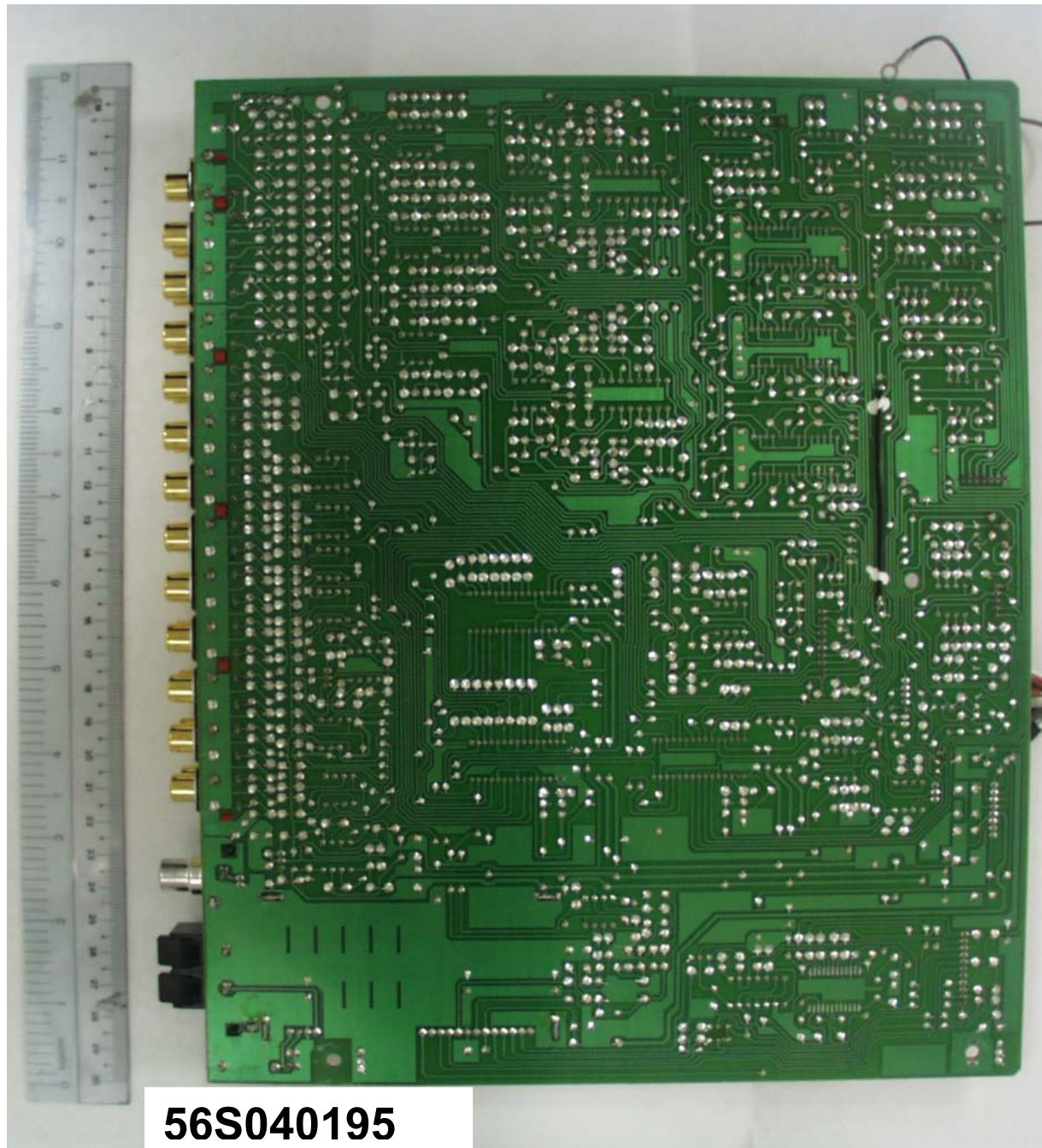
AV Unit – Analog Trace Side
