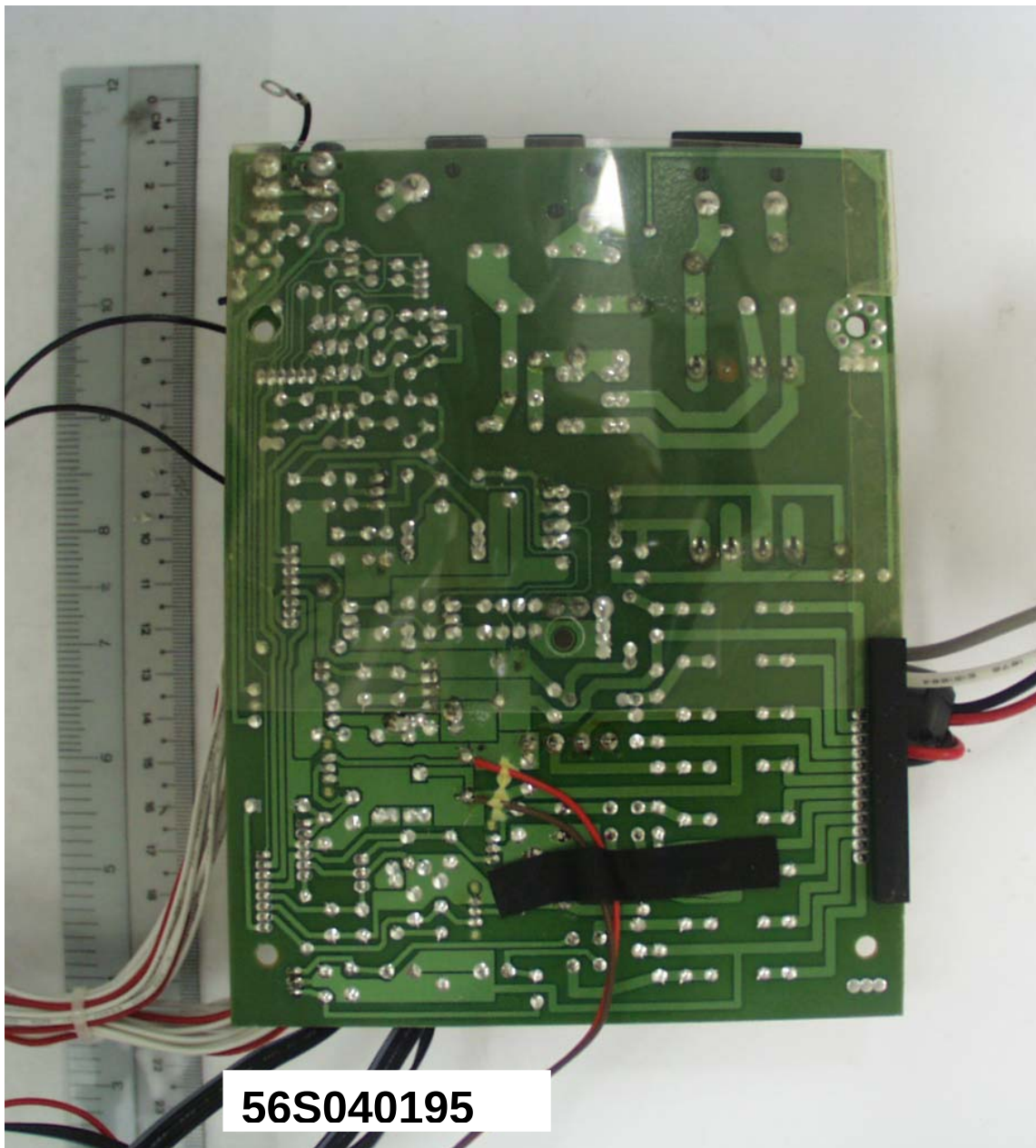
AV Unit – Power Supply Trace Side
