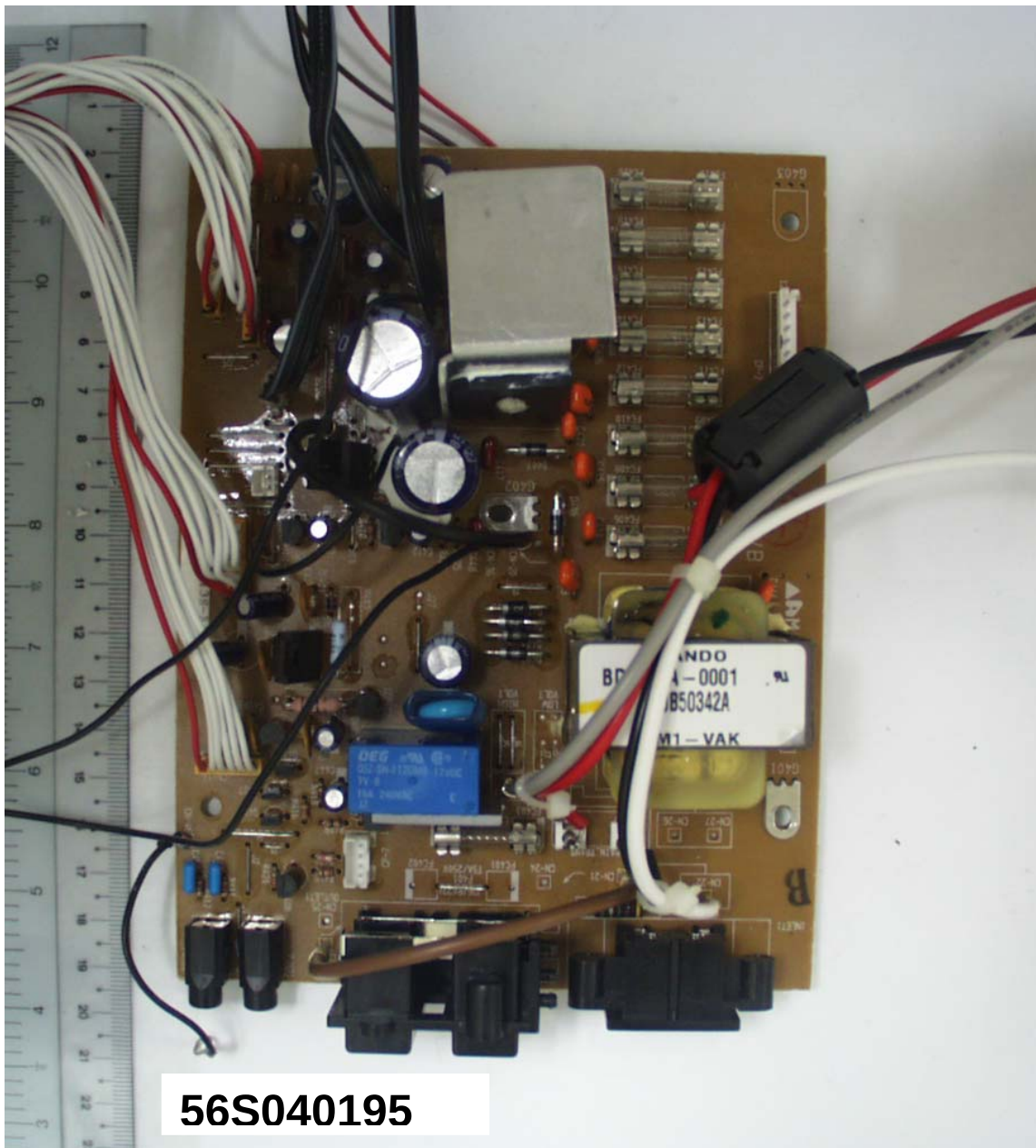
AV Unit – Power Supply Component Side
