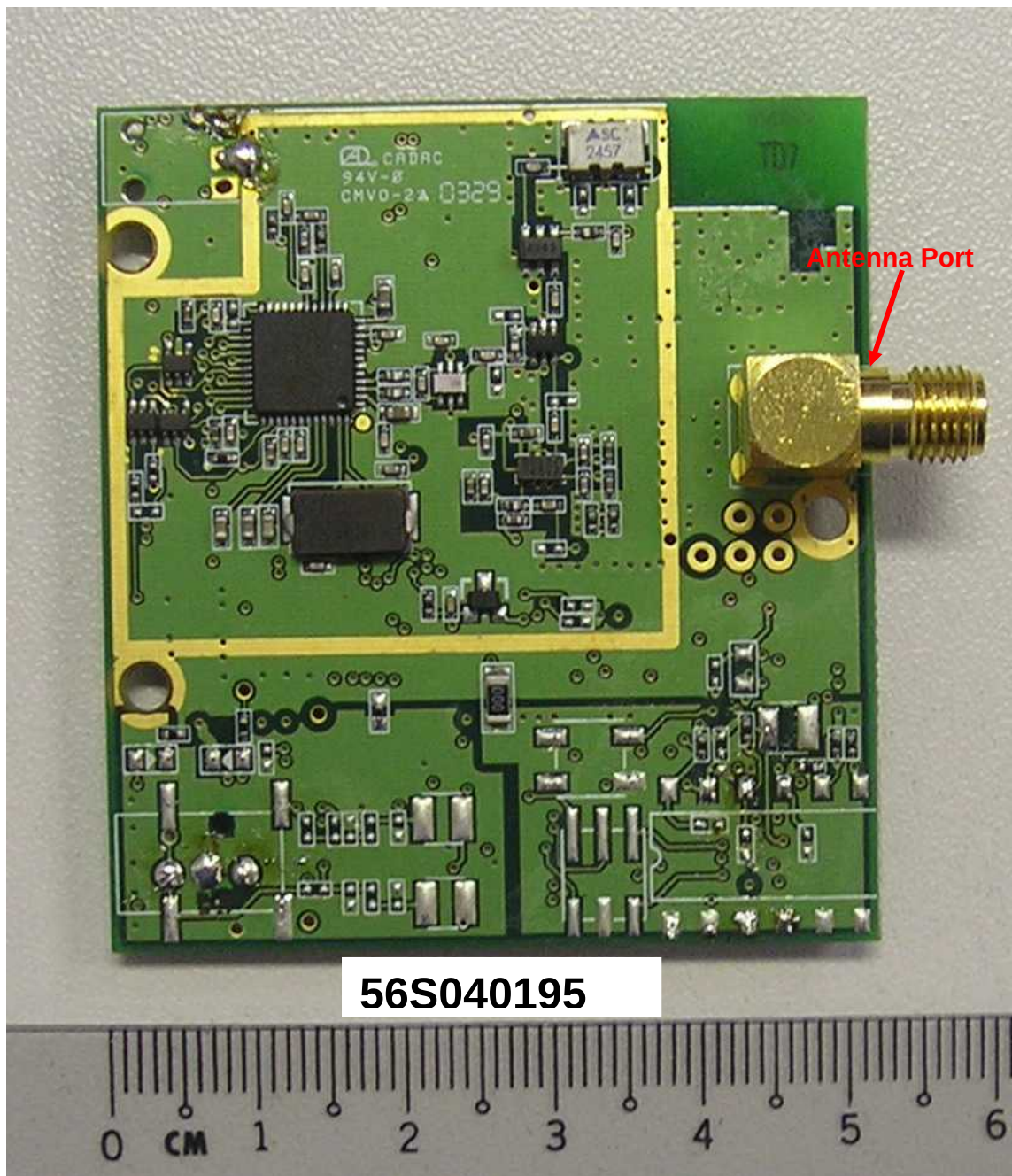
AV Unit – RF Board Trace Side
