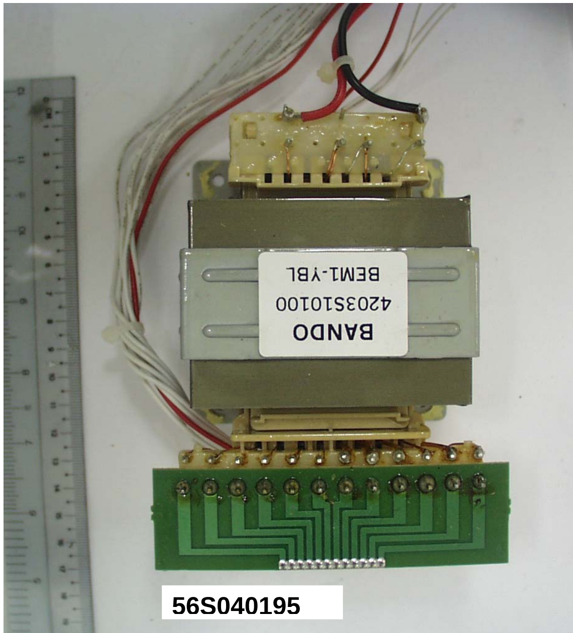
AV Unit – Power Transformer Board Component View 1
