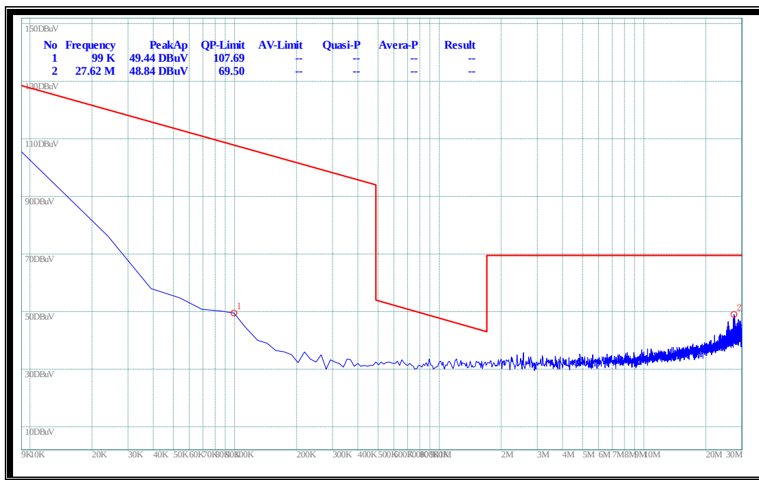
(Plot E.1: 9kHz to 30MHz)
