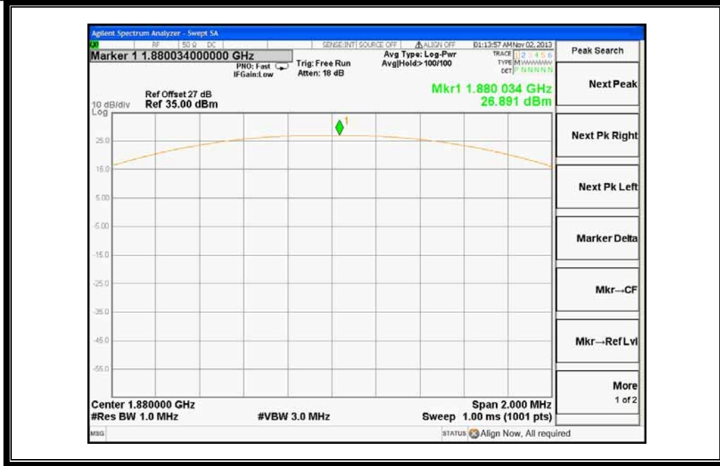
(Plot F2:EGPRS 1900MHz Channel = 661)
