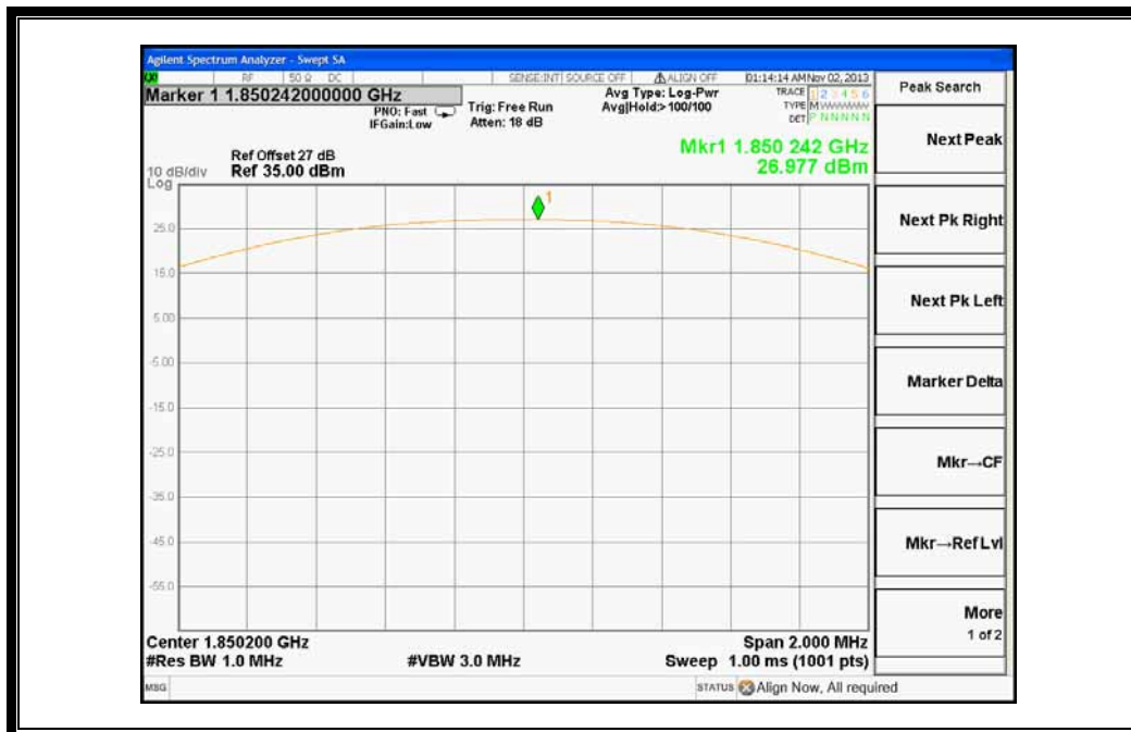
(Plot F1:EGPRS 1900MHz Channel = 512)
