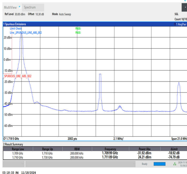
Band66_20MHz_QPSK_132072_1RB#0
