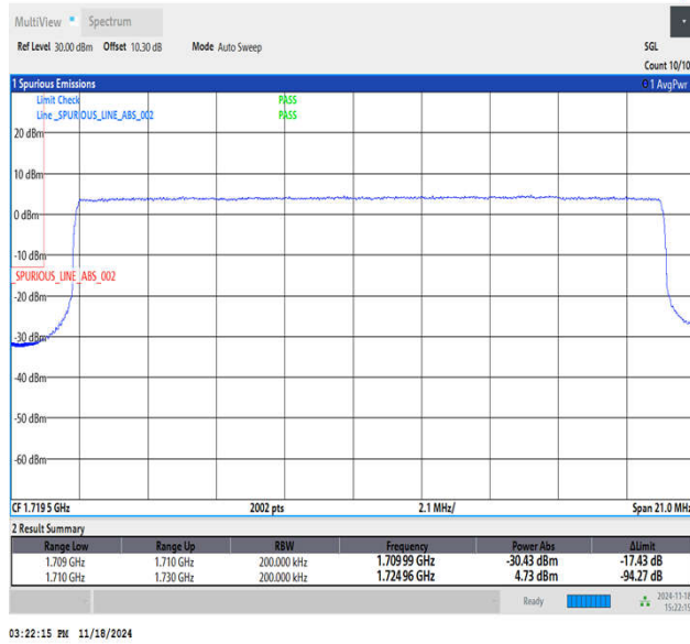
Band66_20MHz_QPSK_132072_100RB#0
