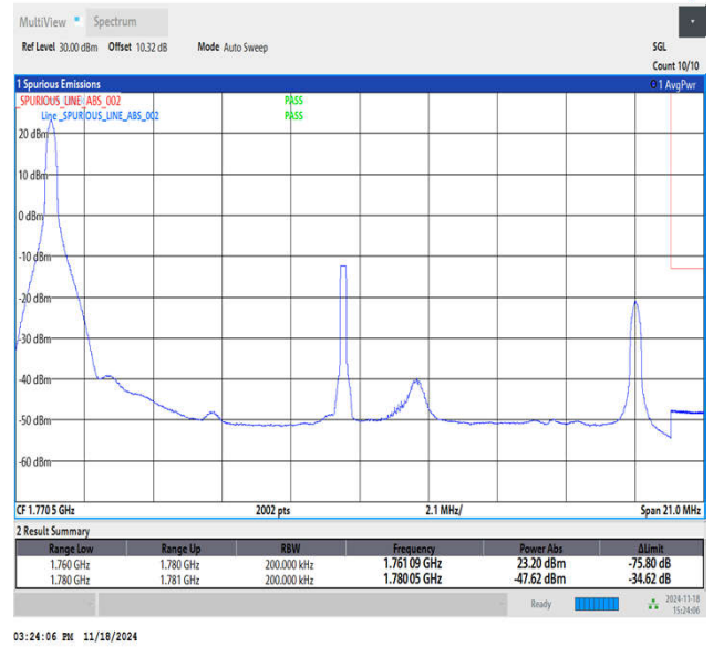
Band66_20MHz_QPSK_132572_1RB#0
