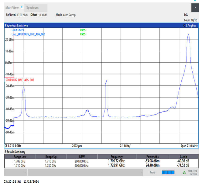
Band66_20MHz_QPSK_132072_1RB#99
