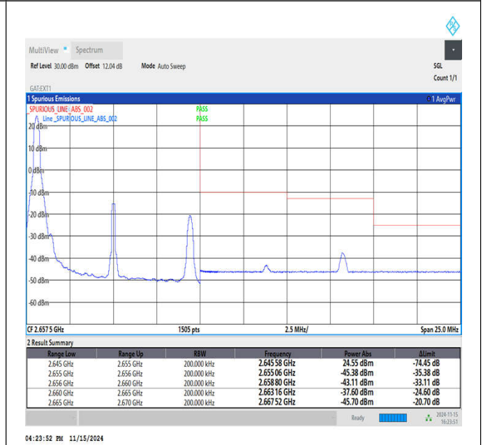
Band41_10MHz_QPSK_41190_1RB#0
