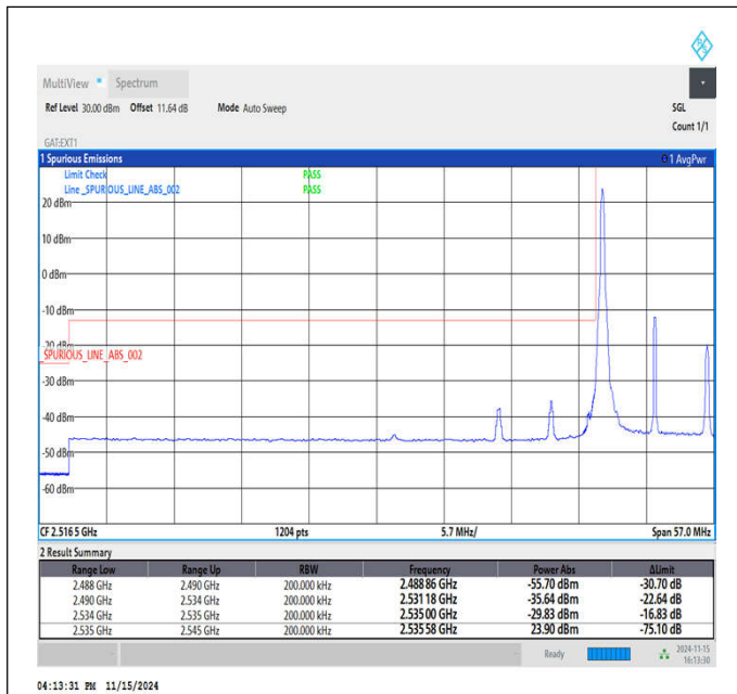
Band41_10MHz_QPSK_40090_1RB#0
