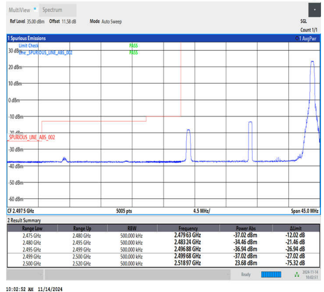
Band7_20MHz_16QAM_20850_1RB#99
