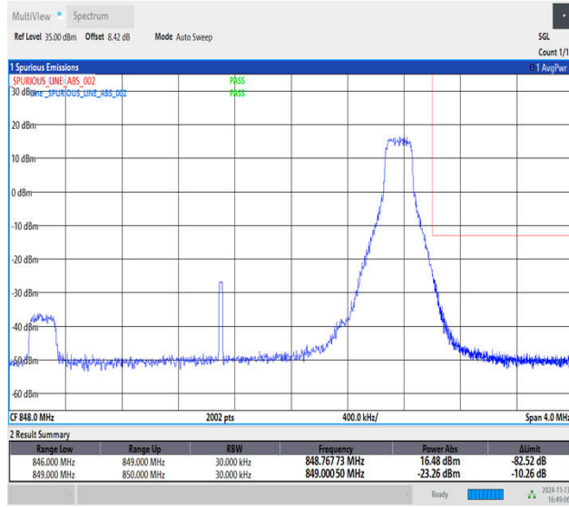
Band5_3MHz_64QAM_20635_1RB#14
