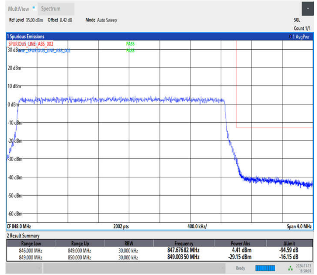
Band5_3MHz_64QAM_20635_15RB#0
