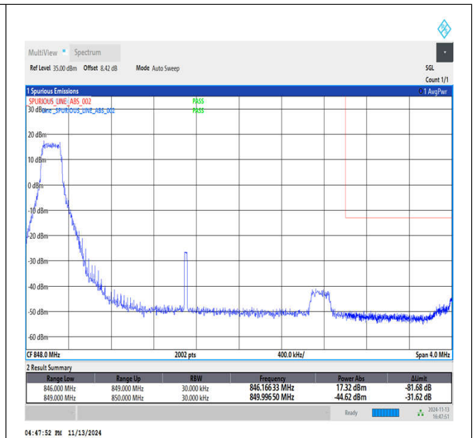
Band5_3MHz_16QAM_20635_1RB#0
