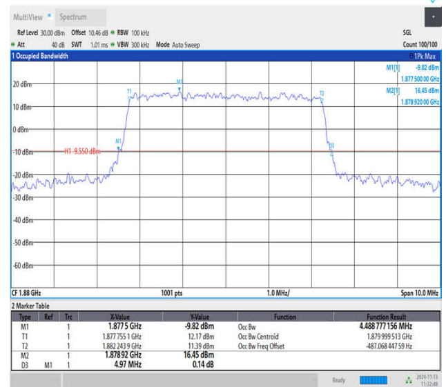
Band2-5MHz-QPSK-18900-25RB#0-PASS
