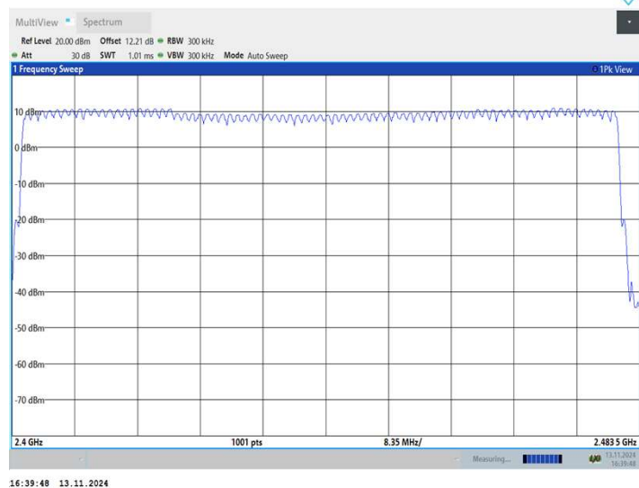
3DH1_Ant1_Hop
