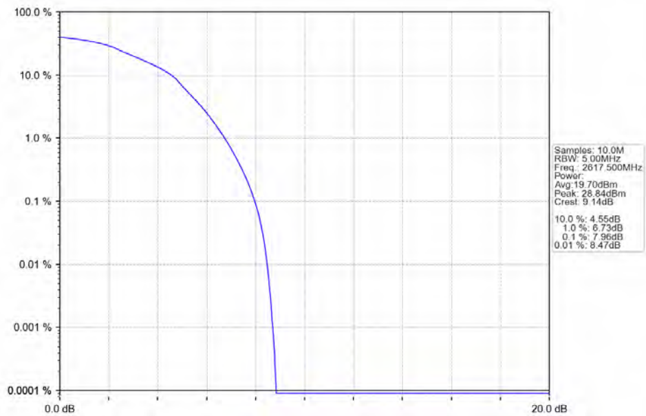
Band38 5MHz 16QAM HCH 2617.5MHz RB 25 0 NTV
